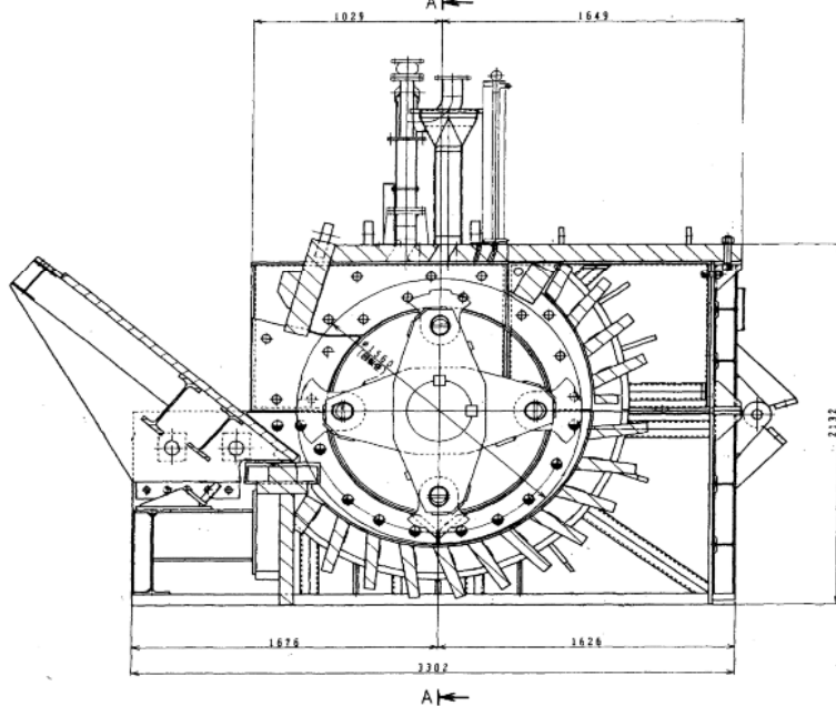
回転破砕機断面図
