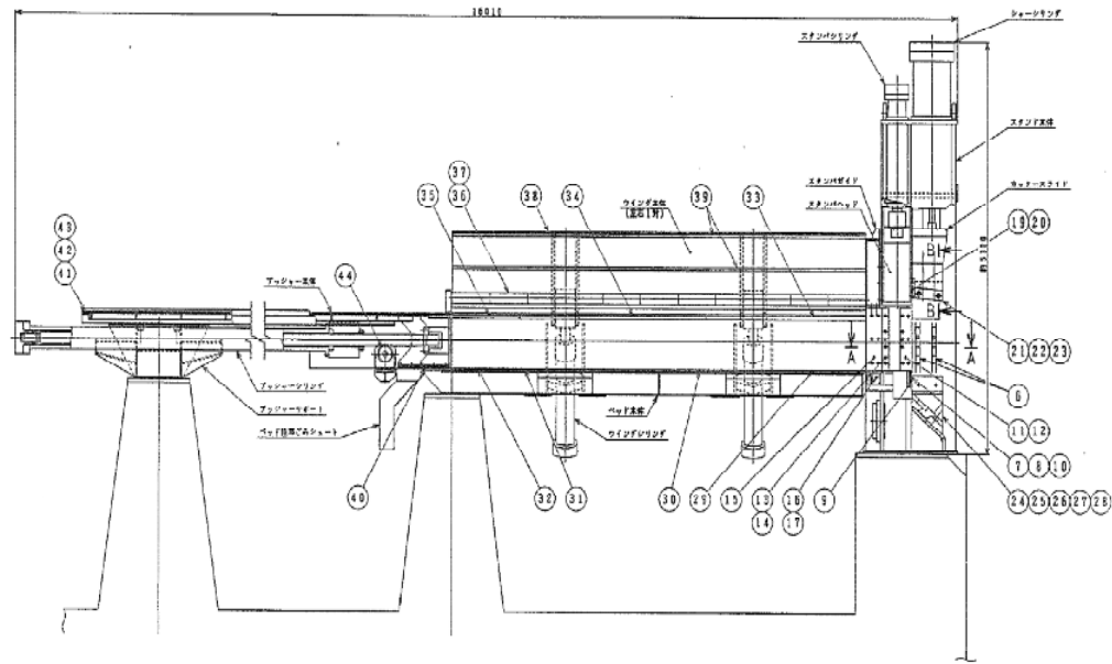
剪断破碎機断面図
