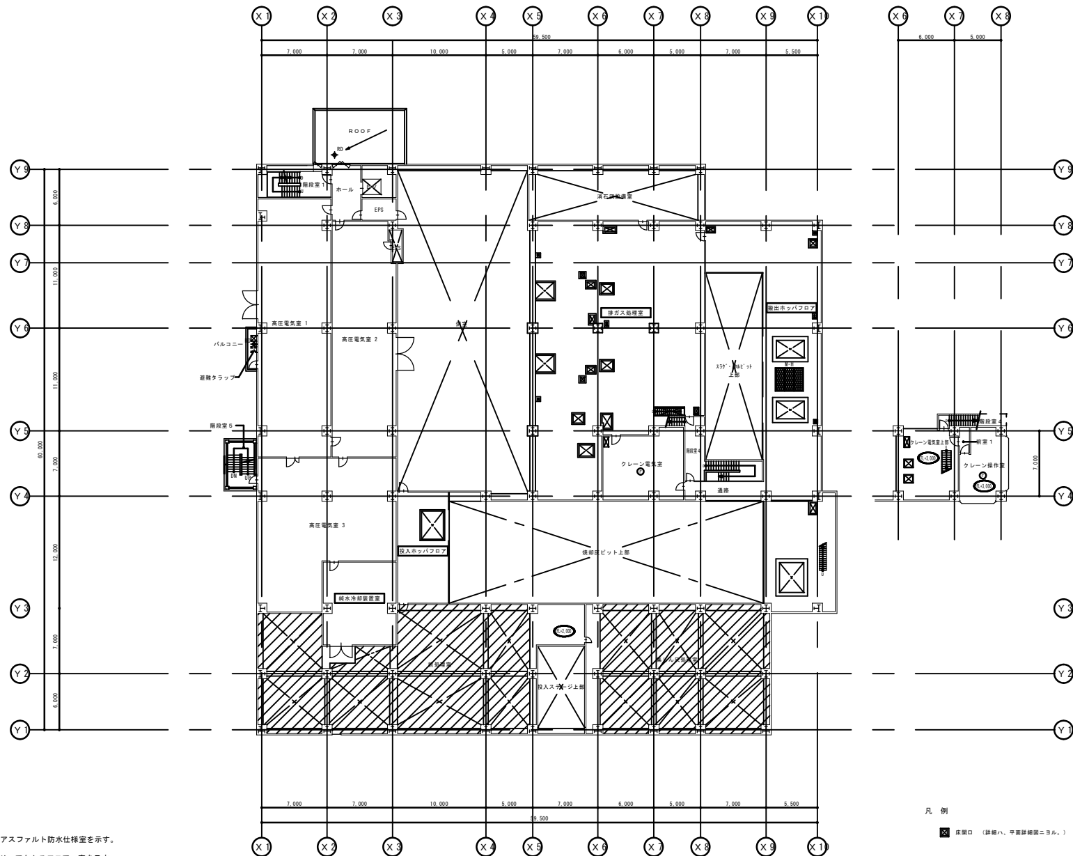
2階平面図 1/200
