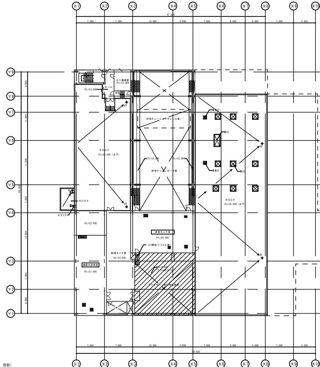
5階平面図 1/200
