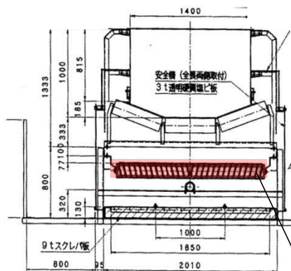
ベルトクリーナ設置図
