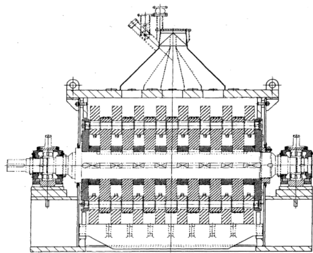
断面 A-A
