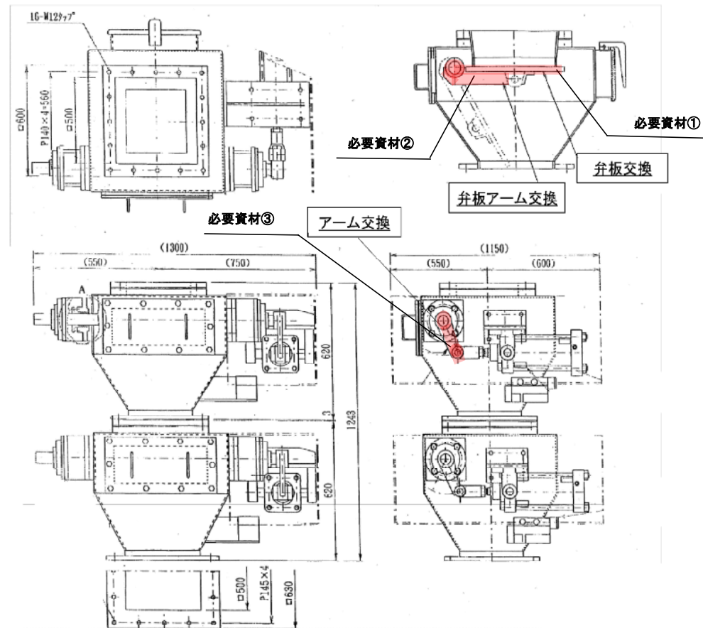
回転系バグフィルタブルダンパ整備
