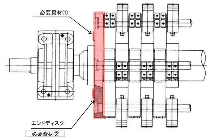
ローター組立図
