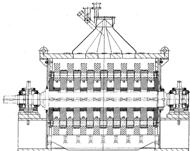
断面A-A
