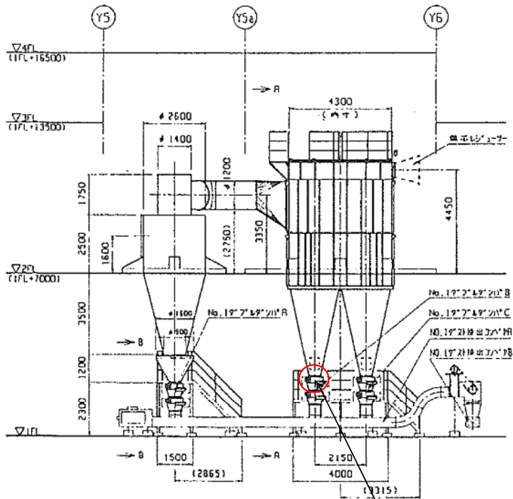
回転系バグフィルタダブルダンパ整備
