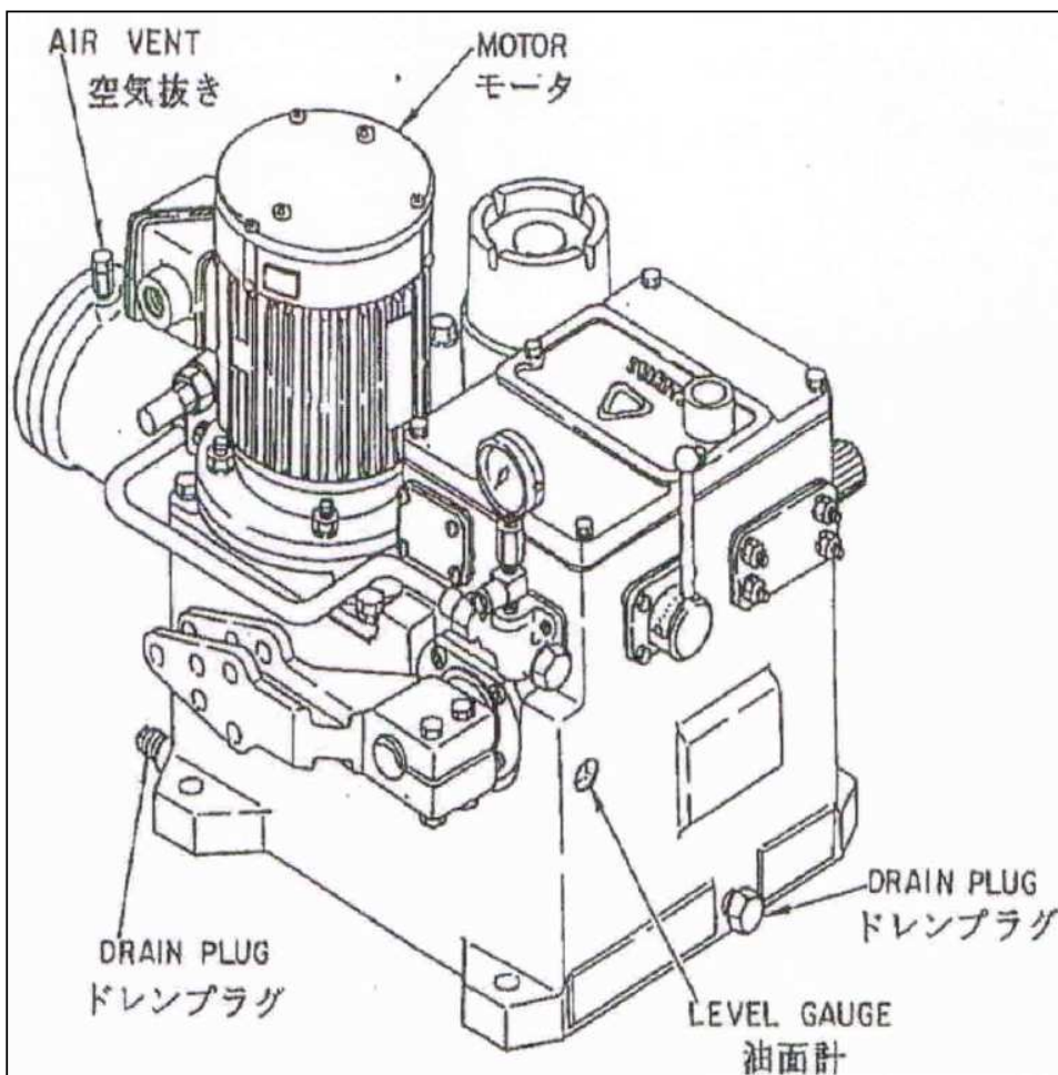
EOP2(SAH燃焼空気温調ダンパ用電油操作器)
