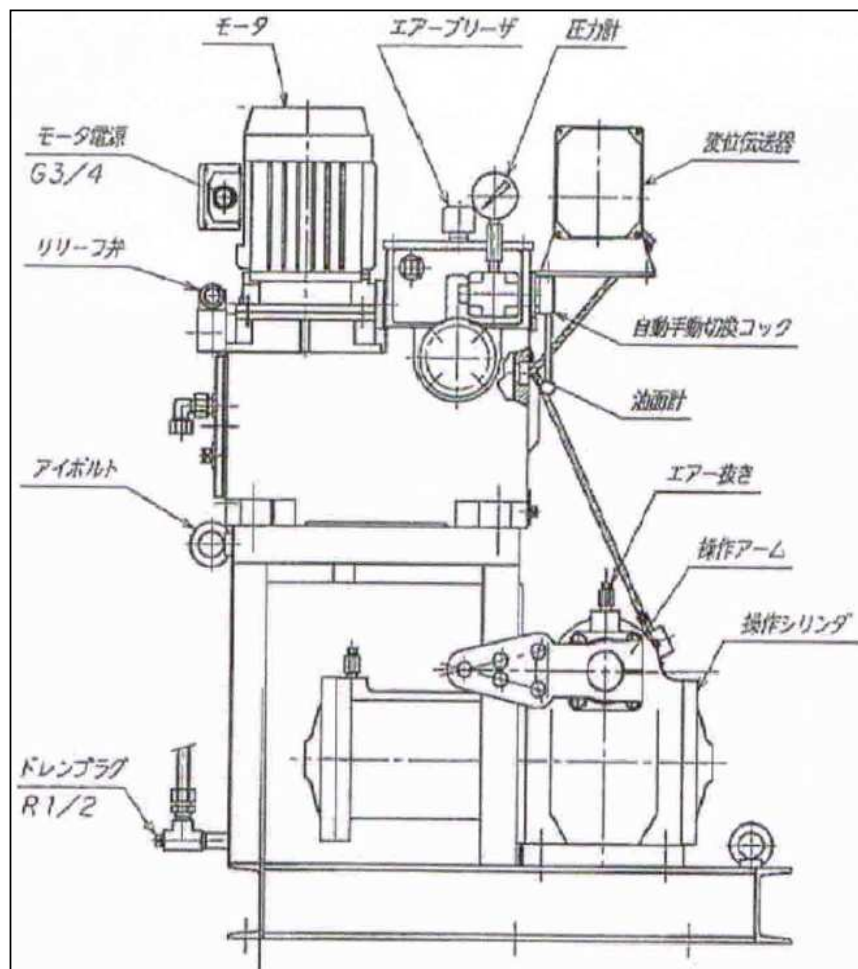
EOP313(炉圧制御ダンパ用電油操作器)
