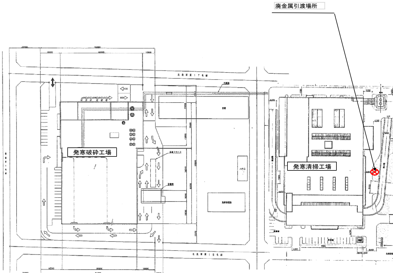
配置図
