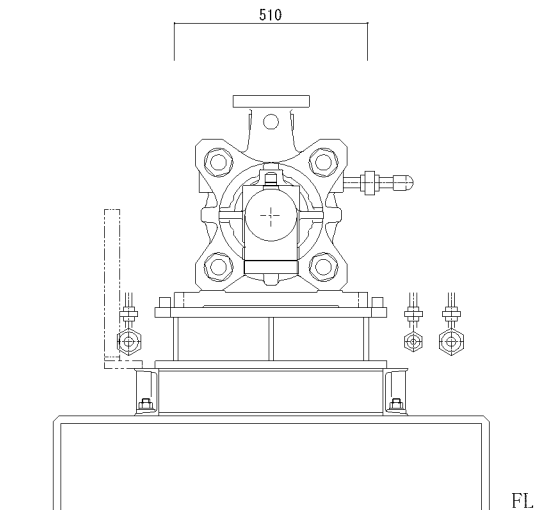
A 矢視図
