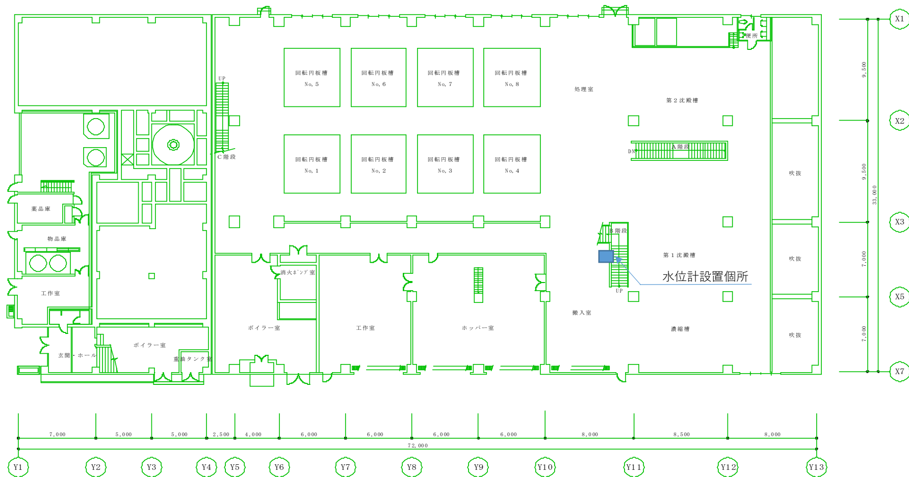
全体 1 階 平面 図
