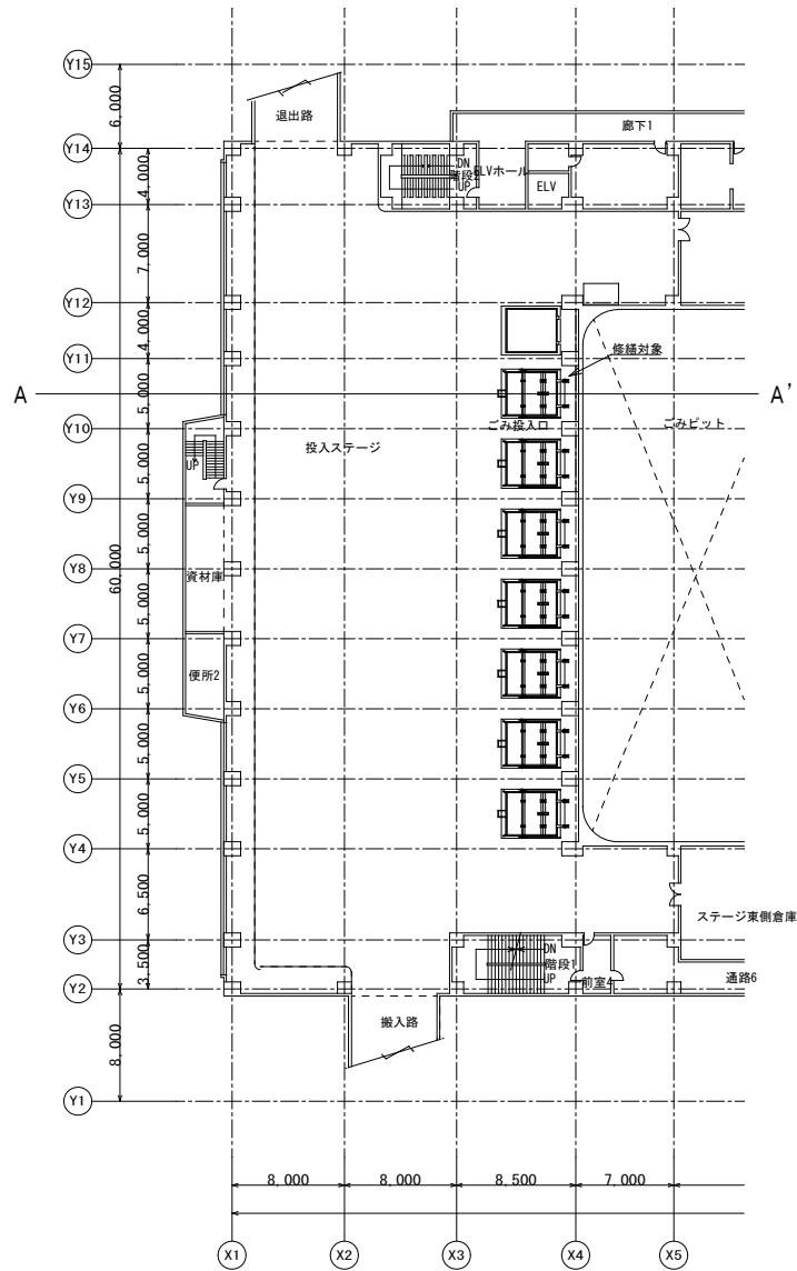
2階 平面図
