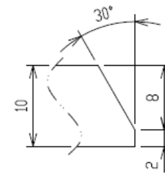
開先B詳細 (SC:NTS)
