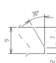
開先A詳細 (SC:NTS)
