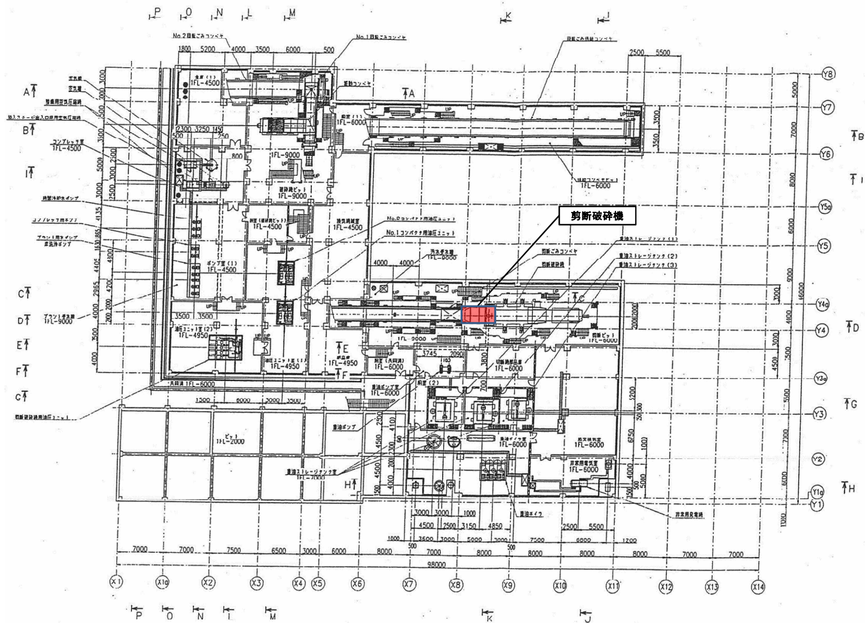
図面名 地階機器配置図 図番 2
