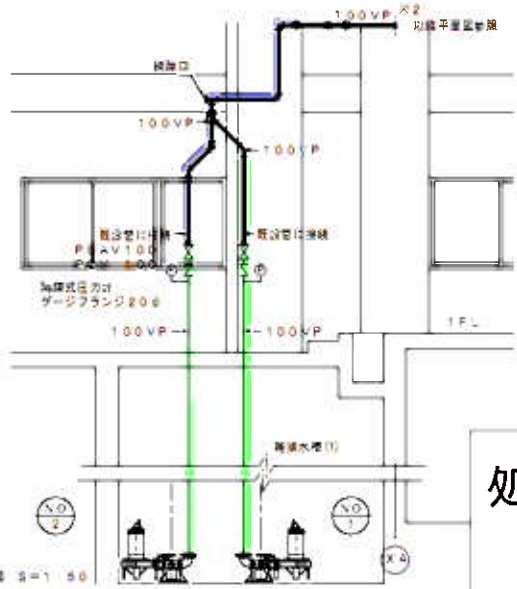
山本北処理施設 断面図 S=1.50
