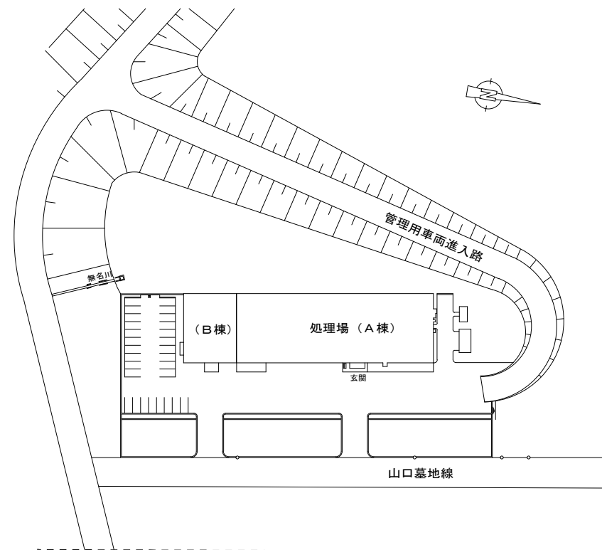
配置図 S=free
