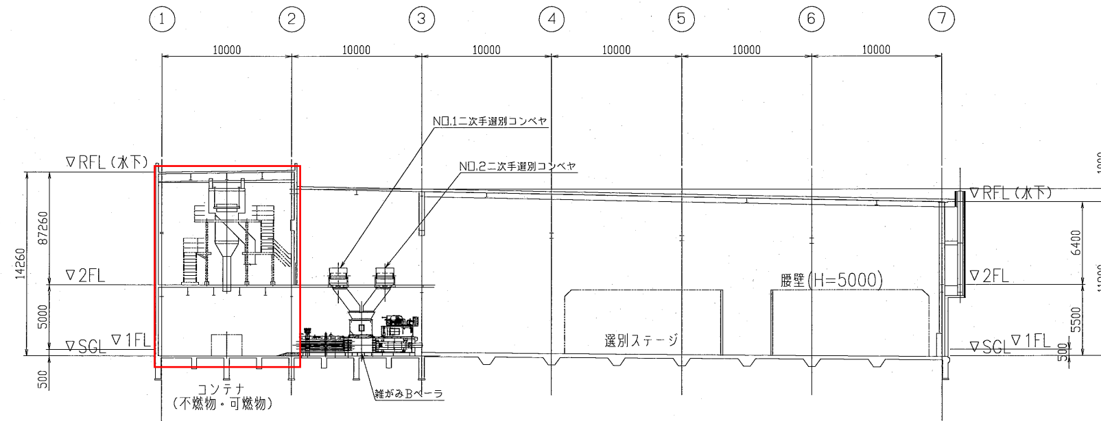
断面A-A
