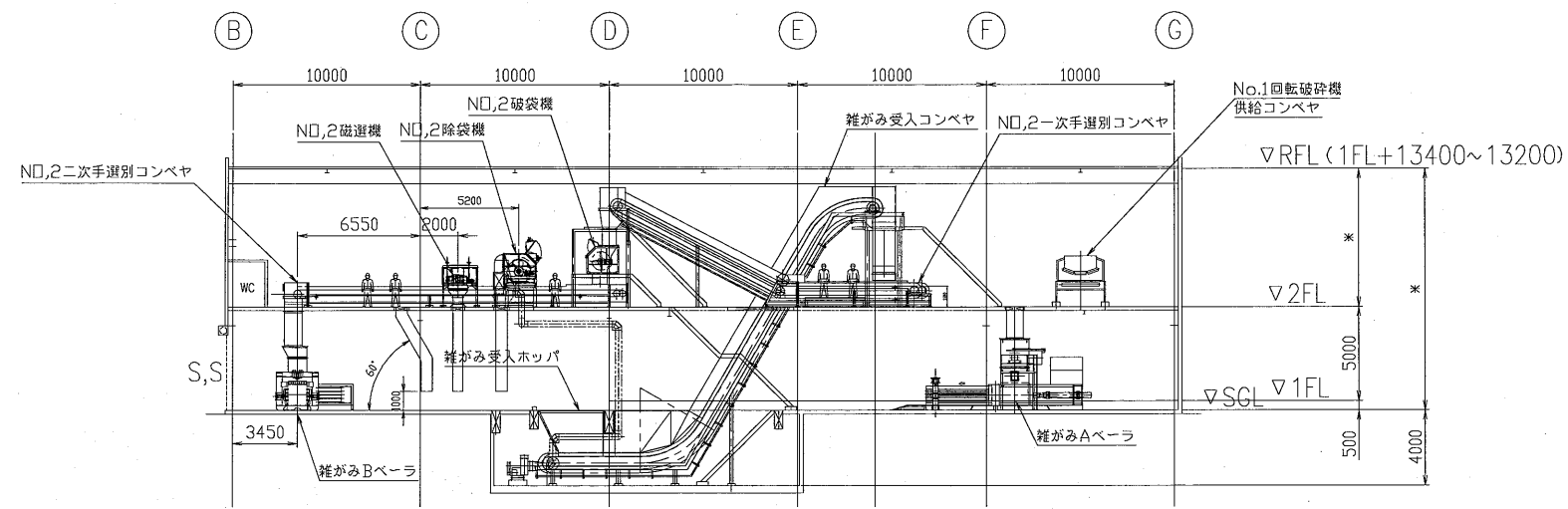
断面B-B
