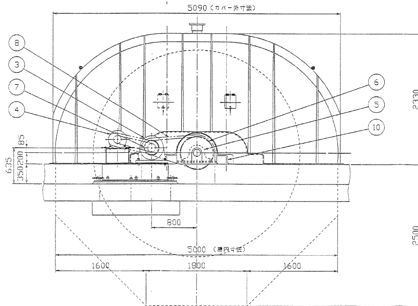
矢視図 A
