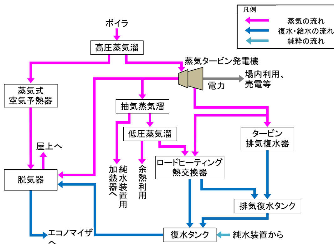
図 2.34 現工場の廃棄物エネルギー利用形態
