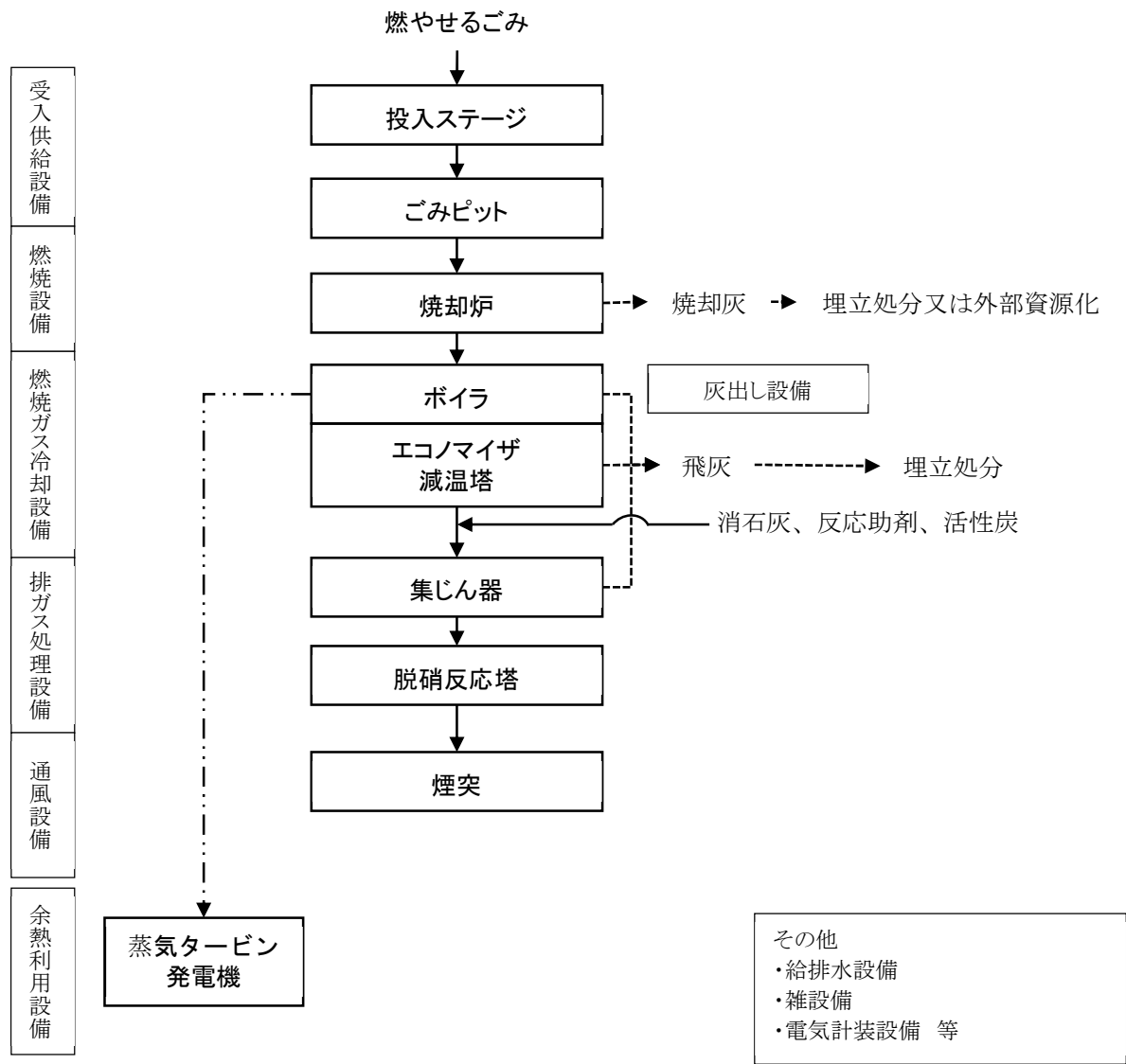
図 2.39 基本処理フロー
