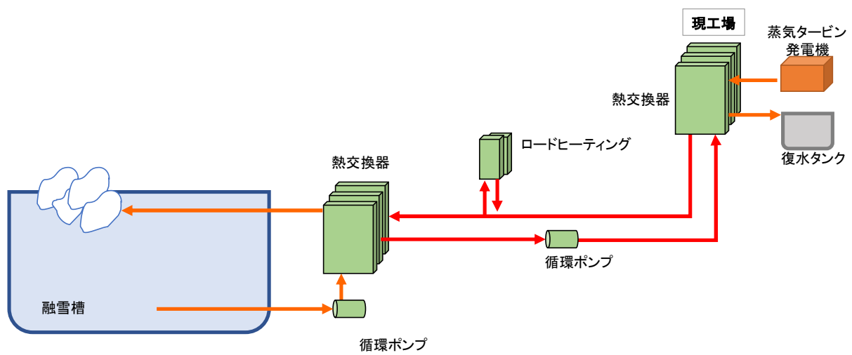
図 2.37 発寒融雪槽の概要図
