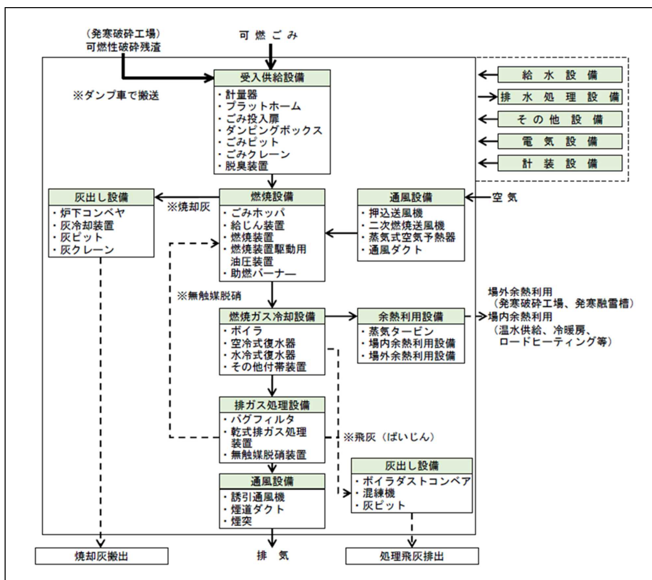
図 8.1 新発寒清掃工場の基本設備構成
