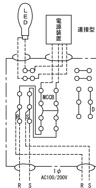
結線図
