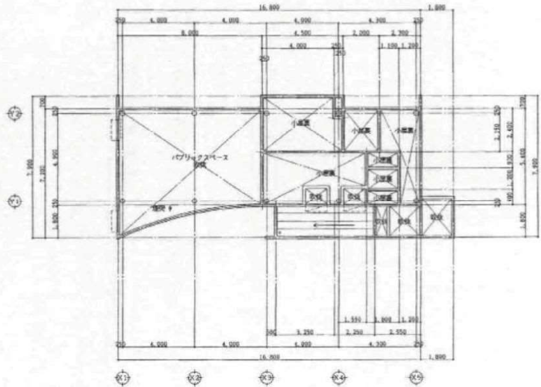
上部平面図
