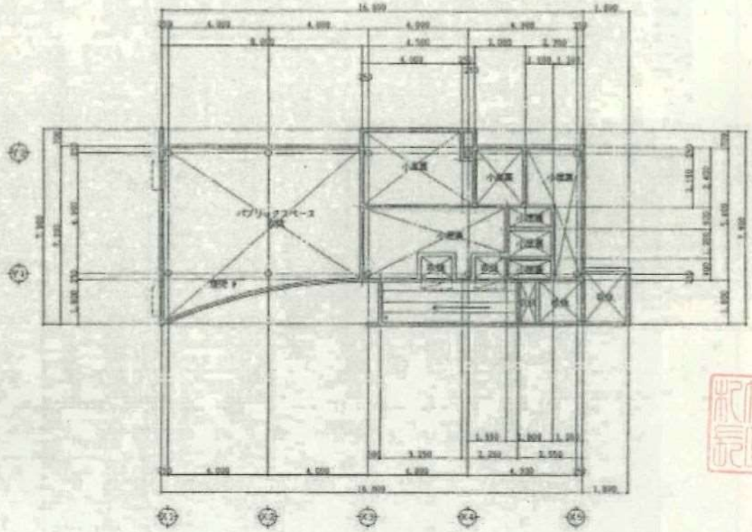
上部平面図
