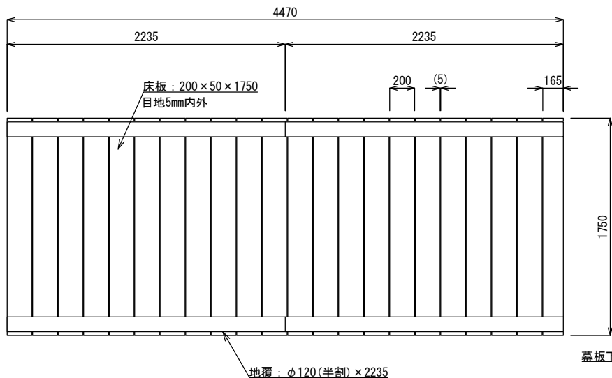
平面図
