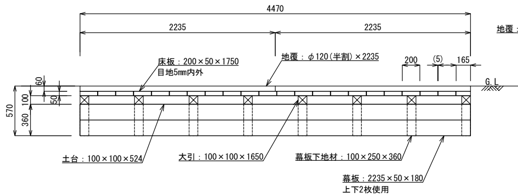
立面図
