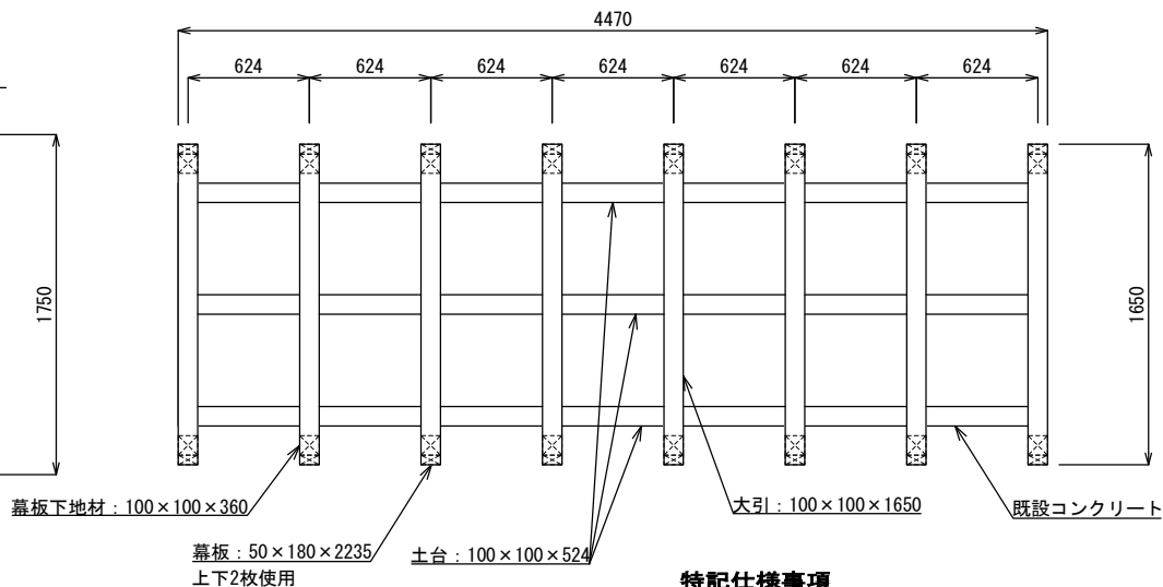
基礎伏図
