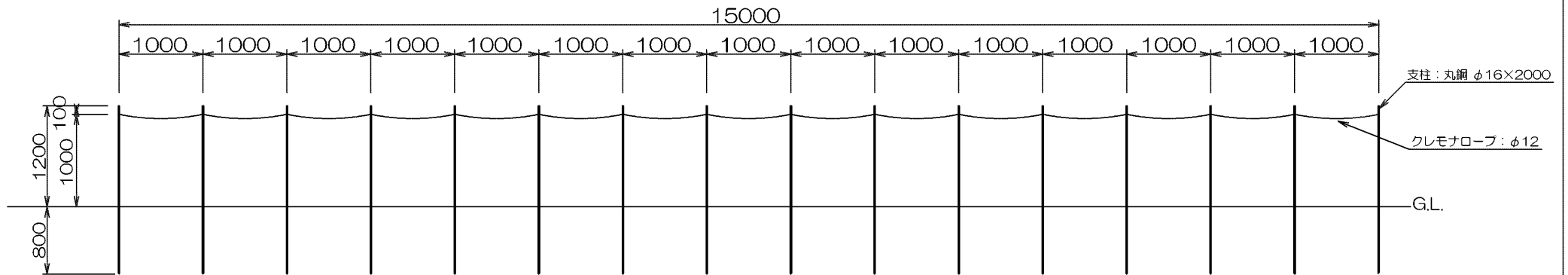
側面図
