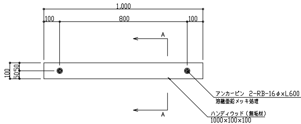
正面図 S=1:10
