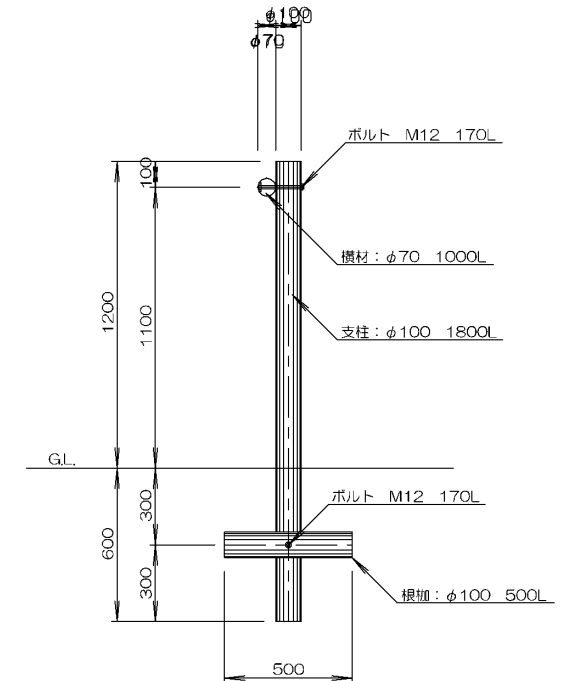
断面図
