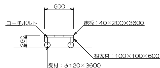
断面図
