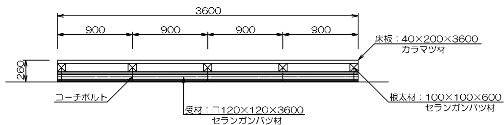
立面図
