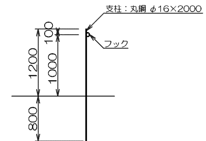
側面図
