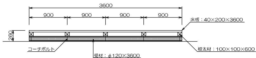
立面図
