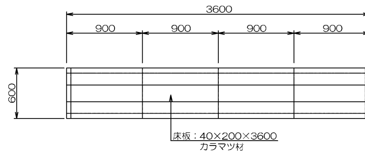
梁伏図
