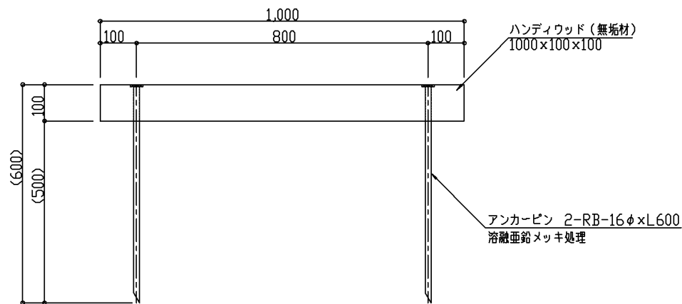
正面図 S=1:10
