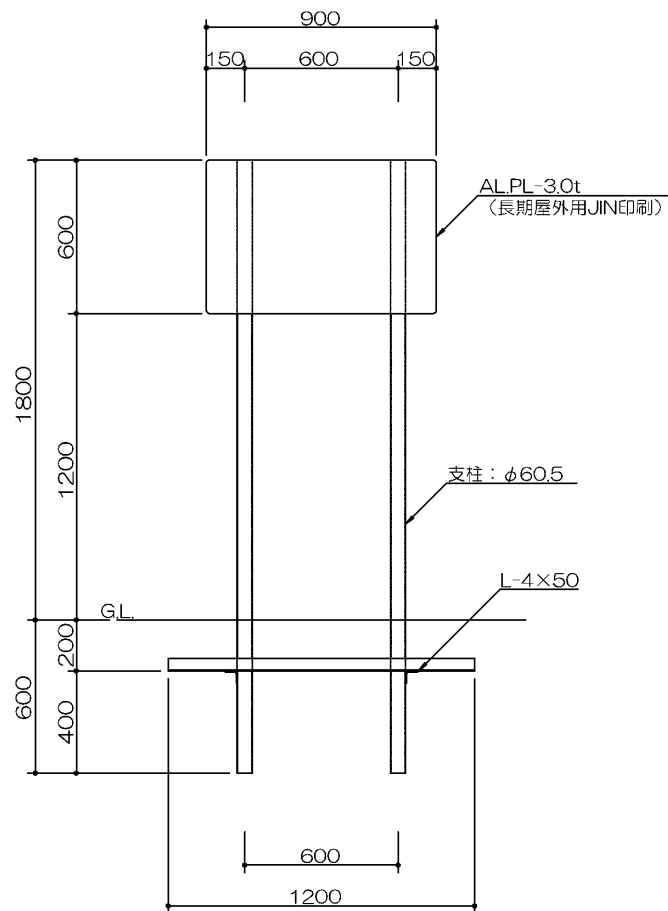
正面図
