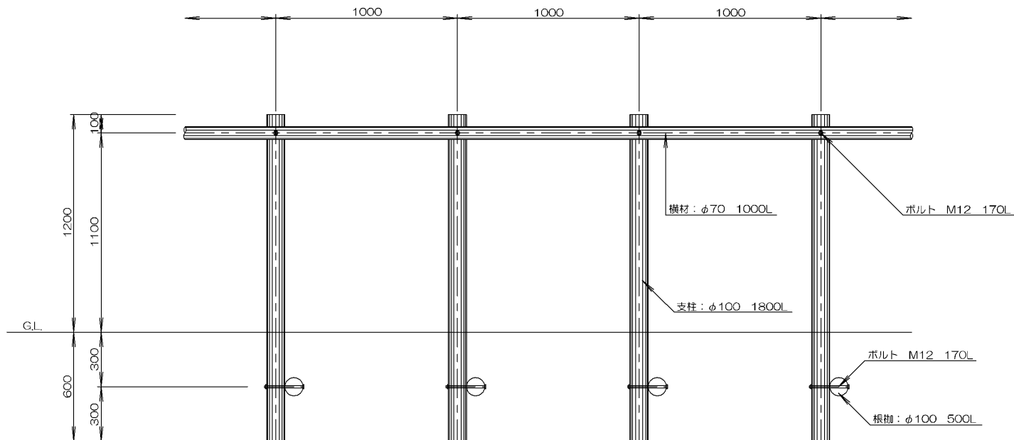
立面図
