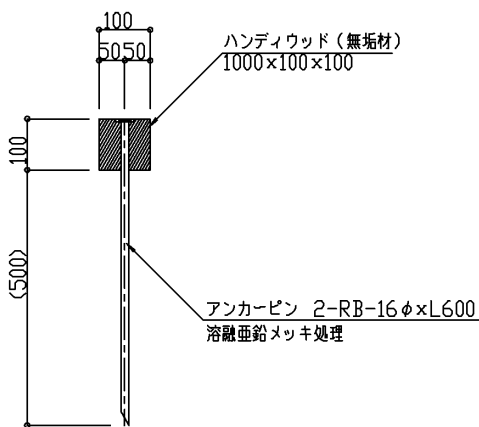
A-A断面図 S=1:10
