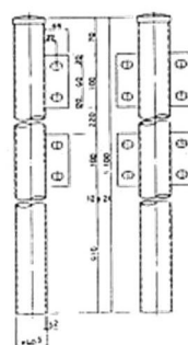
端柱 詳細図
