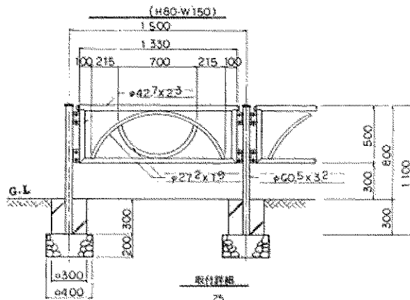
端柱 詳細図 中間柱 詳細図
