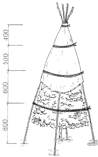
根入部寸法
