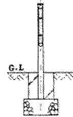
外柵設置図 (W=1.5m) PG-1.5C 又は同等品以上
