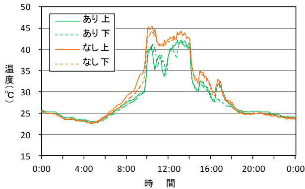
図4 新川保育園での測定結果(平成23年7月29日 左:温度、右:照度) あり:緑のカーテンあり なし:緑のカーテンなし
