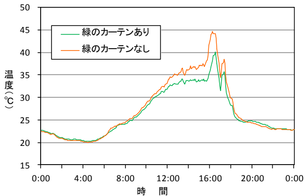
図2 「にじいろ」での測定結果(平成23年7月29日 左:温度、右:照度)
