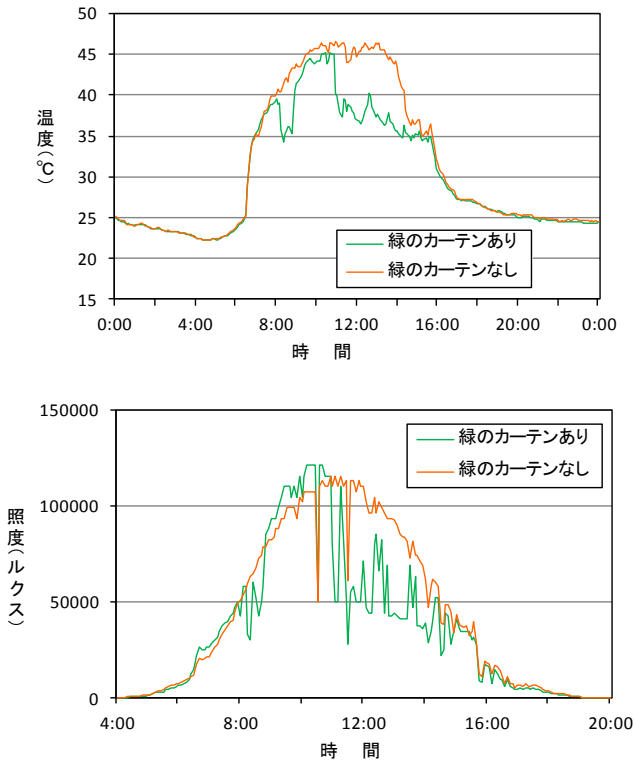
図3 中央図書館での測定結果(平成23年7月29日 上:温度、下:照度)
