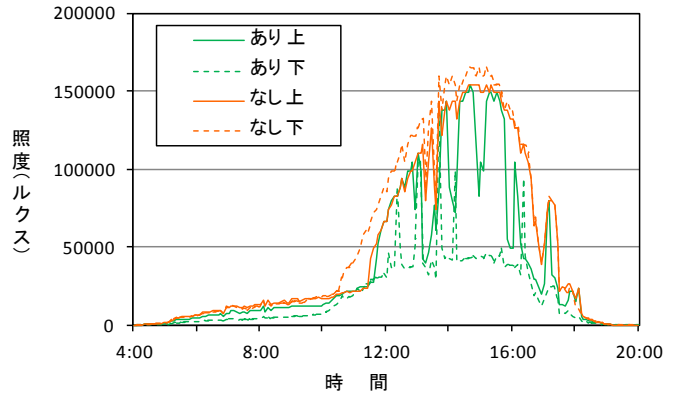
図1 清田区土木センターでの測定結果(平成23年7月29日 左:温度、右:照度)
