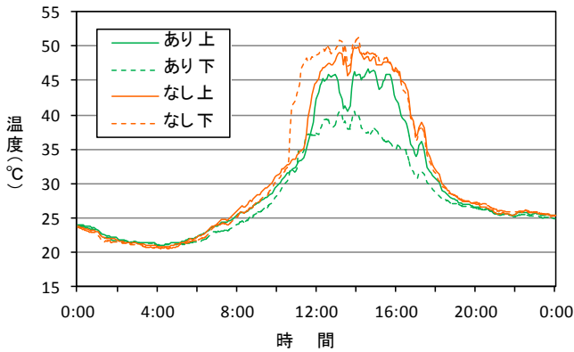
図1 清田区土木センターでの測定結果(平成23年7月29日 左:温度、右:照度)
