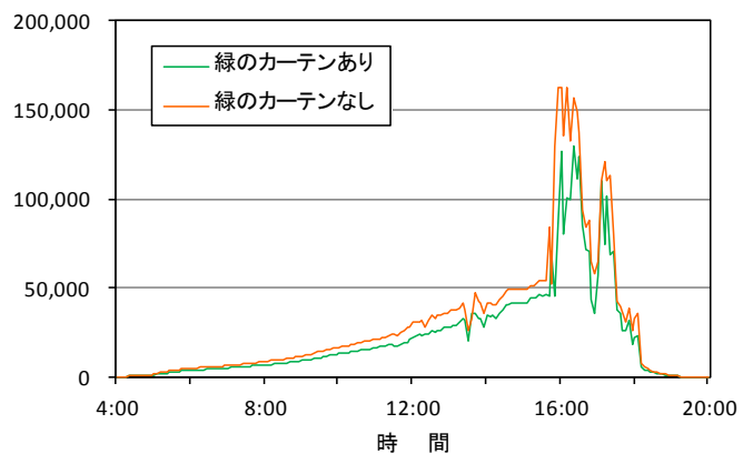
図2 「にじいろ」での測定結果(平成23年7月29日 左:温度、右:照度)
