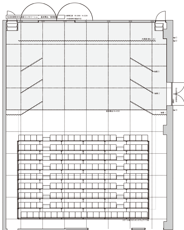
《基本舞台・客席図面》
