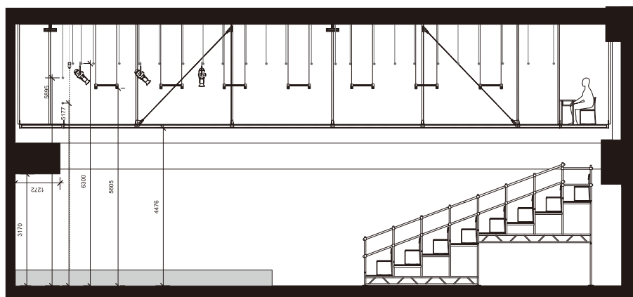
《劇場断面図》
