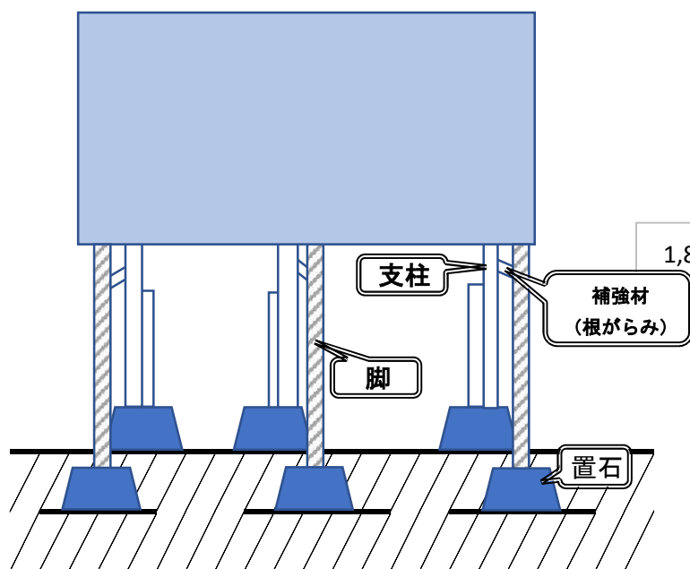
&lt; 正面図 &gt;
