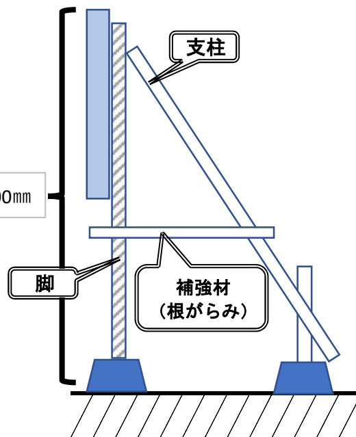
&lt; 側面図 &gt;
