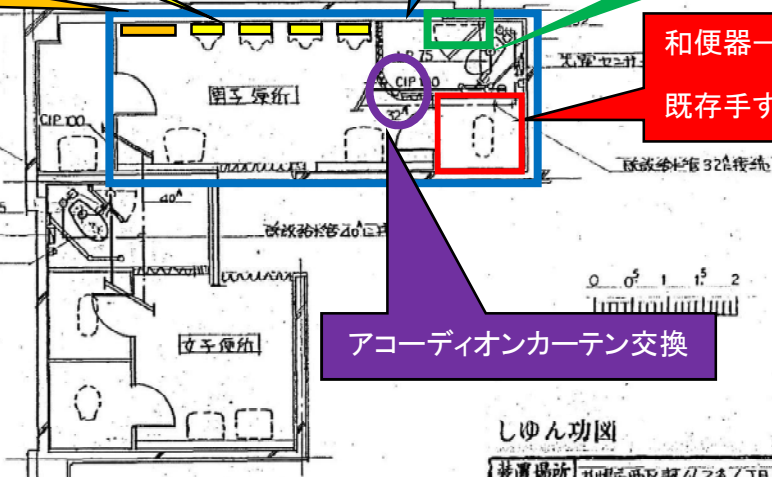
平面図(改修後) S=1/50
