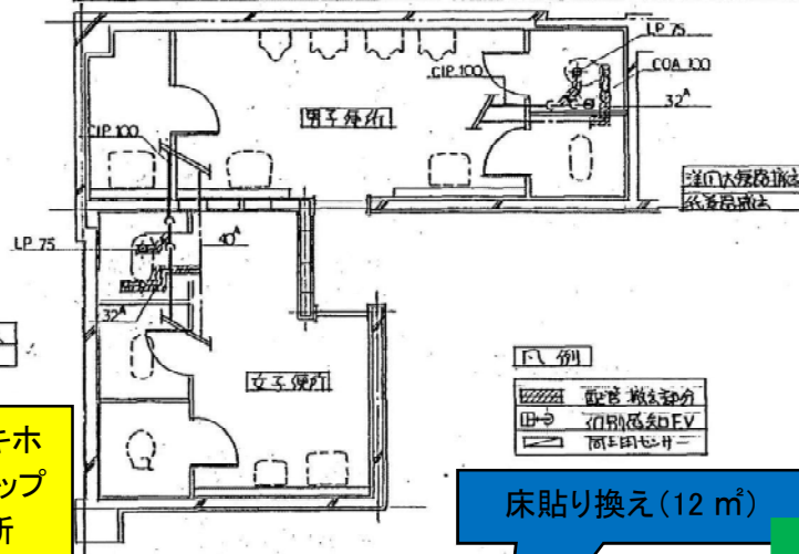
平面図(改修前) S=1/50
