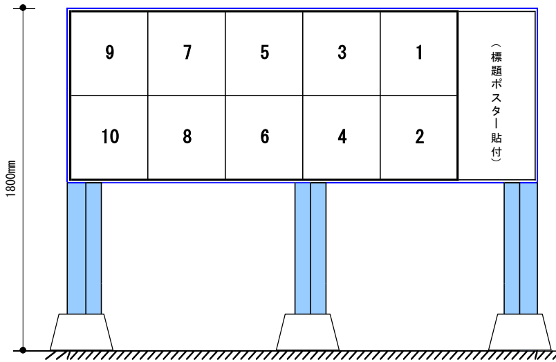
(正面図)
