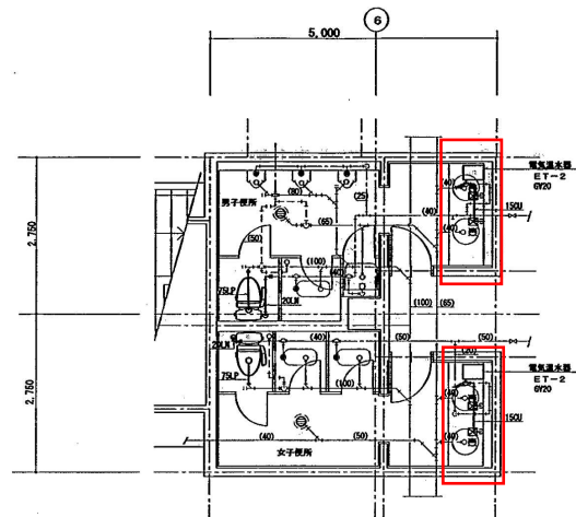
1階 便所詳細図 (衛生設備) S=1/50
