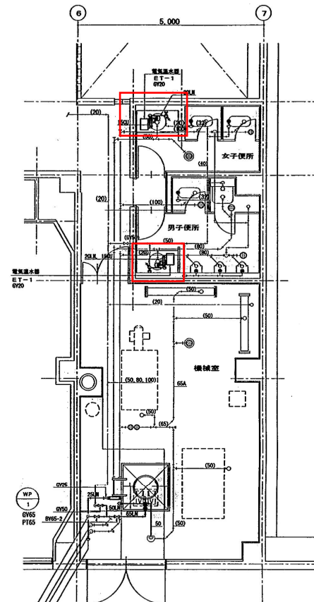
2階 機械室詳細図 (衛生設備) S=1/50
