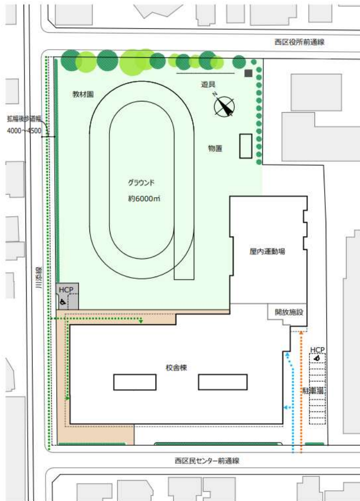
配置図 S=1/800
