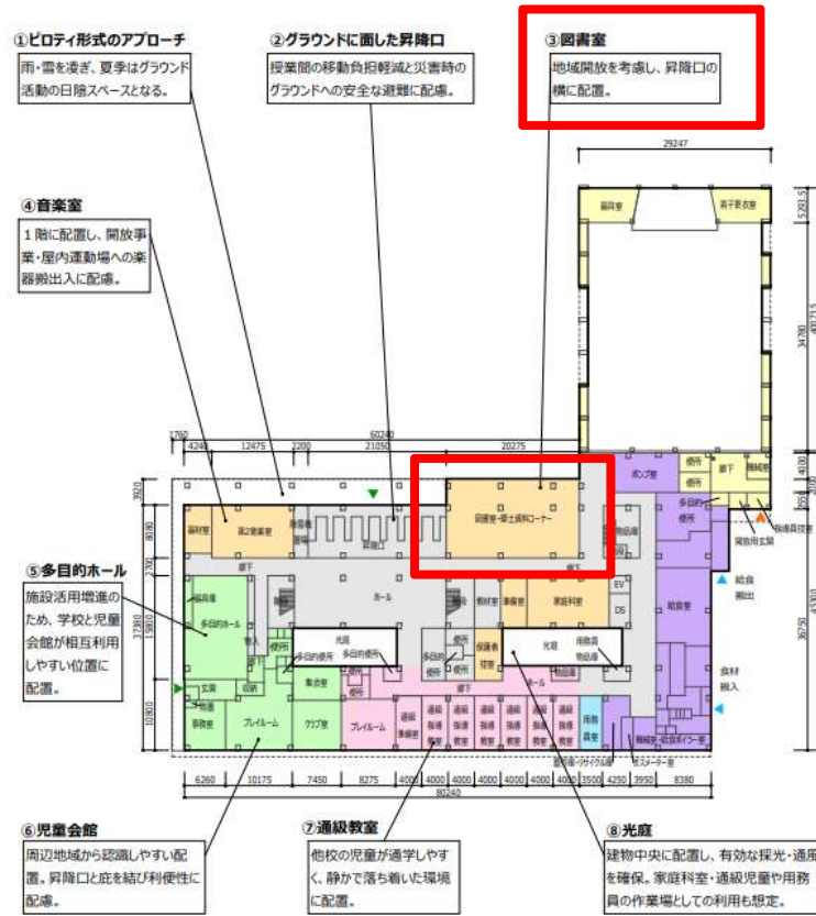
■ 1階平面図
