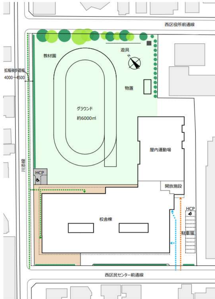
配置図 S=1/800 ▼ 学校・児童会館出入口 ▼ 地域開放出入口 ▼ 搬出入出入口 ●●● 児童動線 ●●● 地域開放動線 ●●● 車両動線
