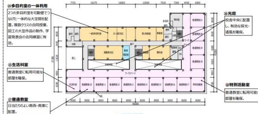
■ 3階平面図
