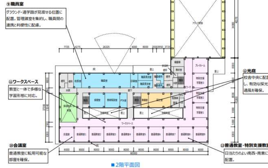
■ 2階平面図
