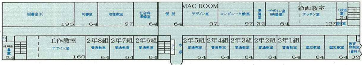
3階平面図
