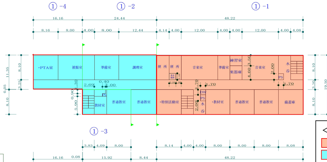
3階平面図
