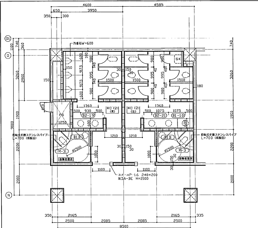
WC (2) 詳細図 (1階~4階)
