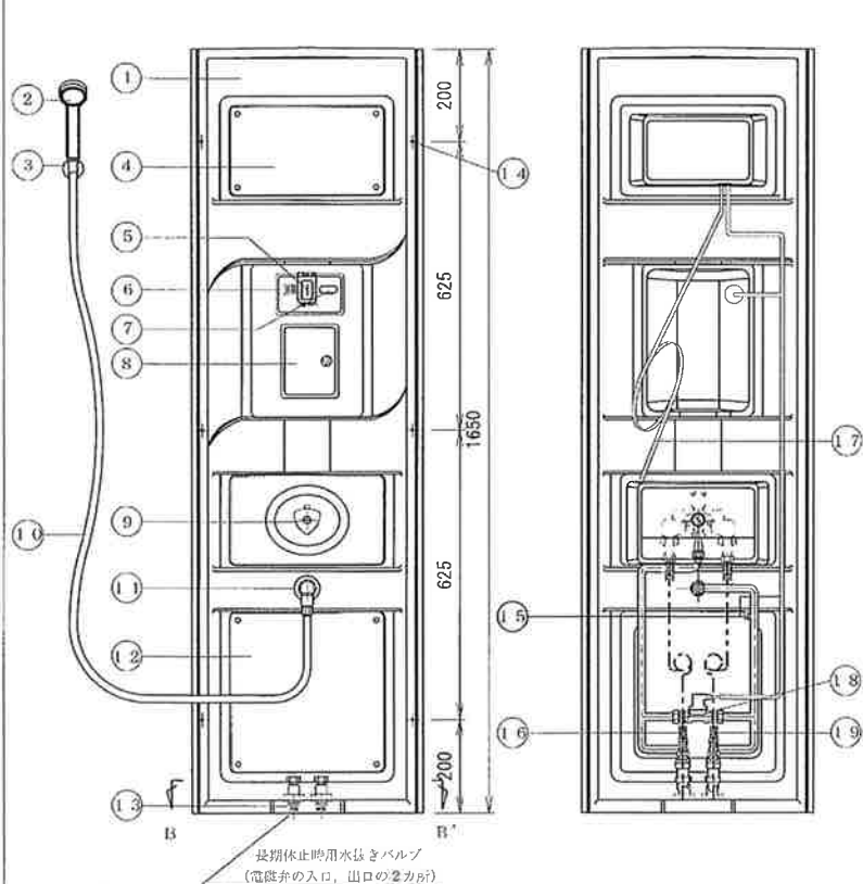
正面図
