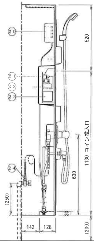
A-A' 断面図
