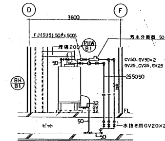
機械室配管断面図 S=1/50
