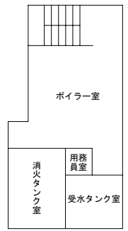
地階平面図
