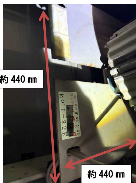
従動側ブラケット
