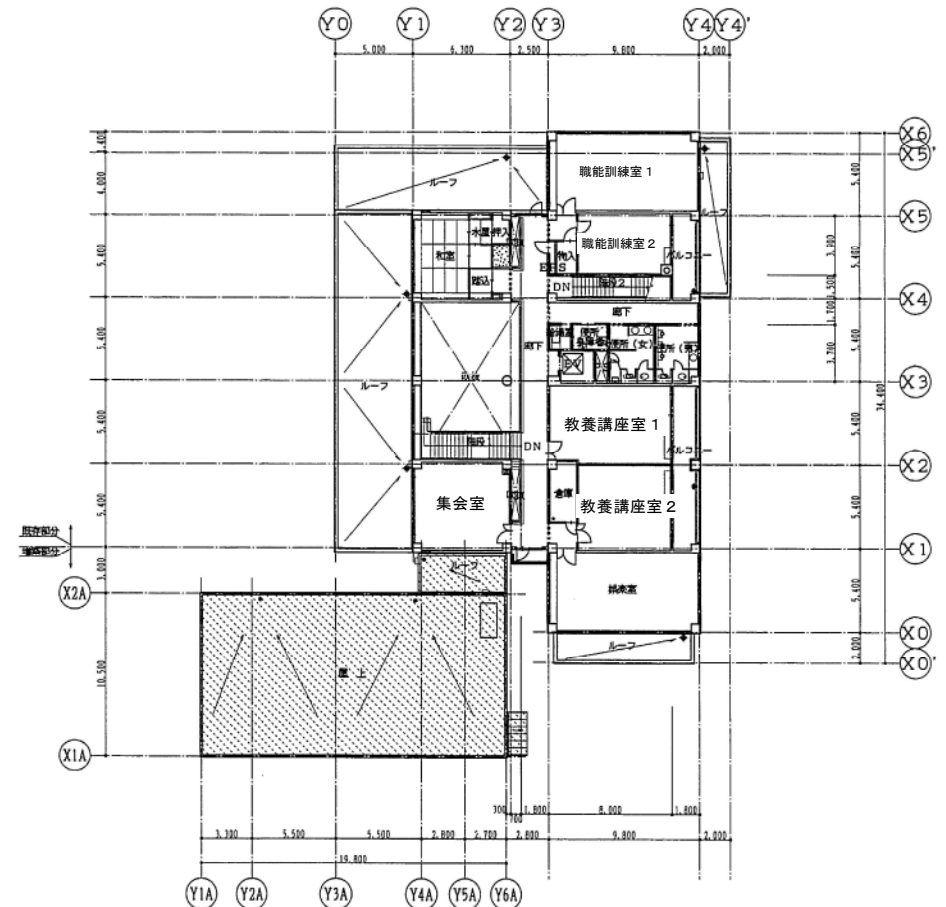
2階平面図 1/200
