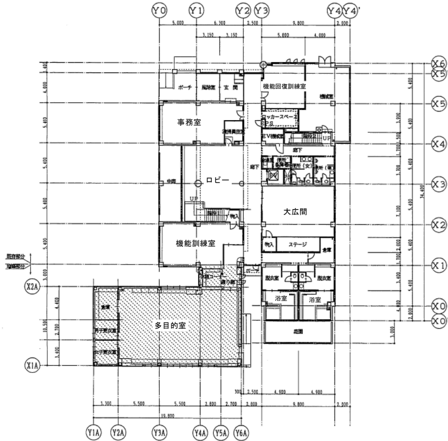
1階平面図 1/200
