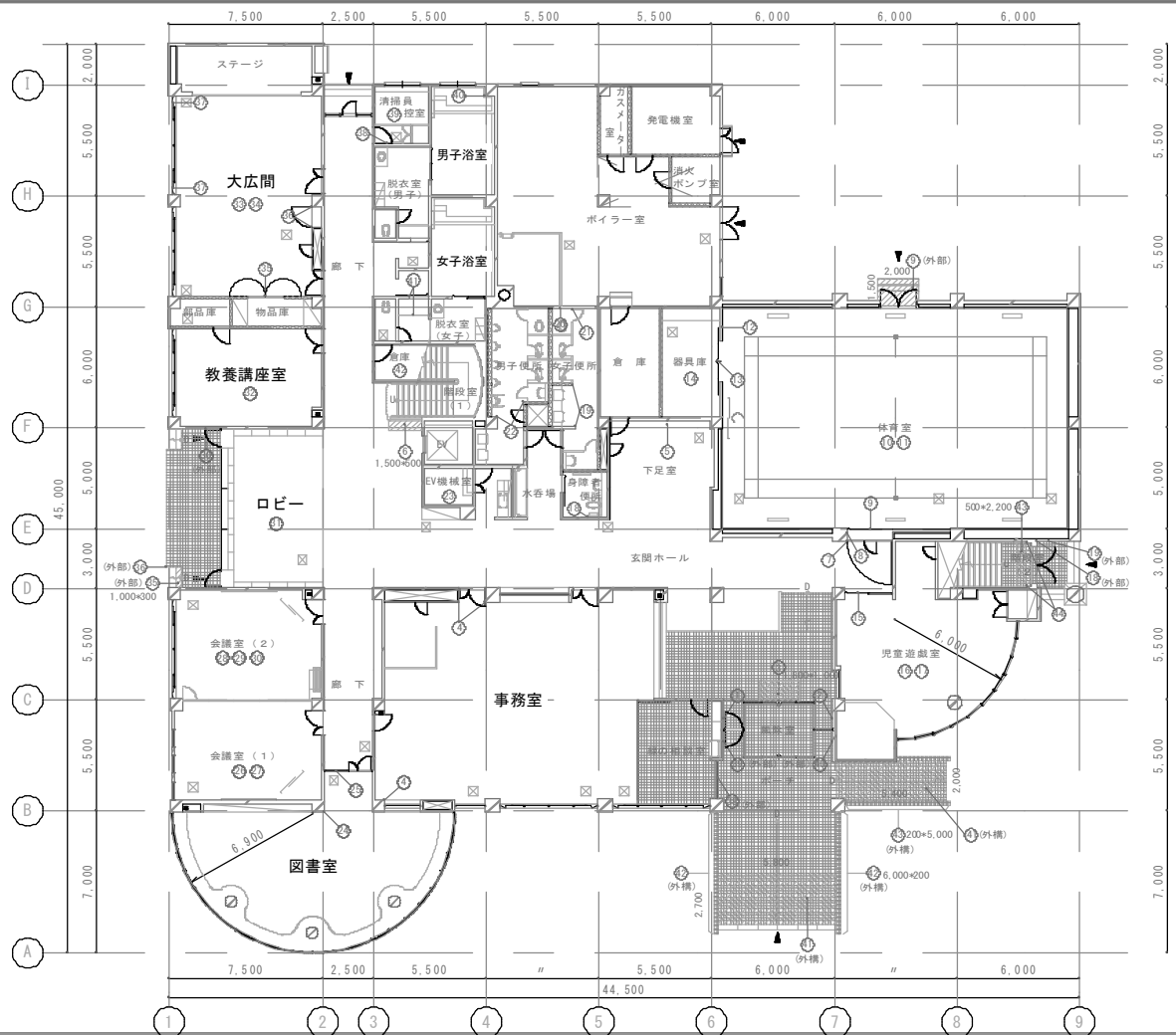
1階平面図 S 1/200
