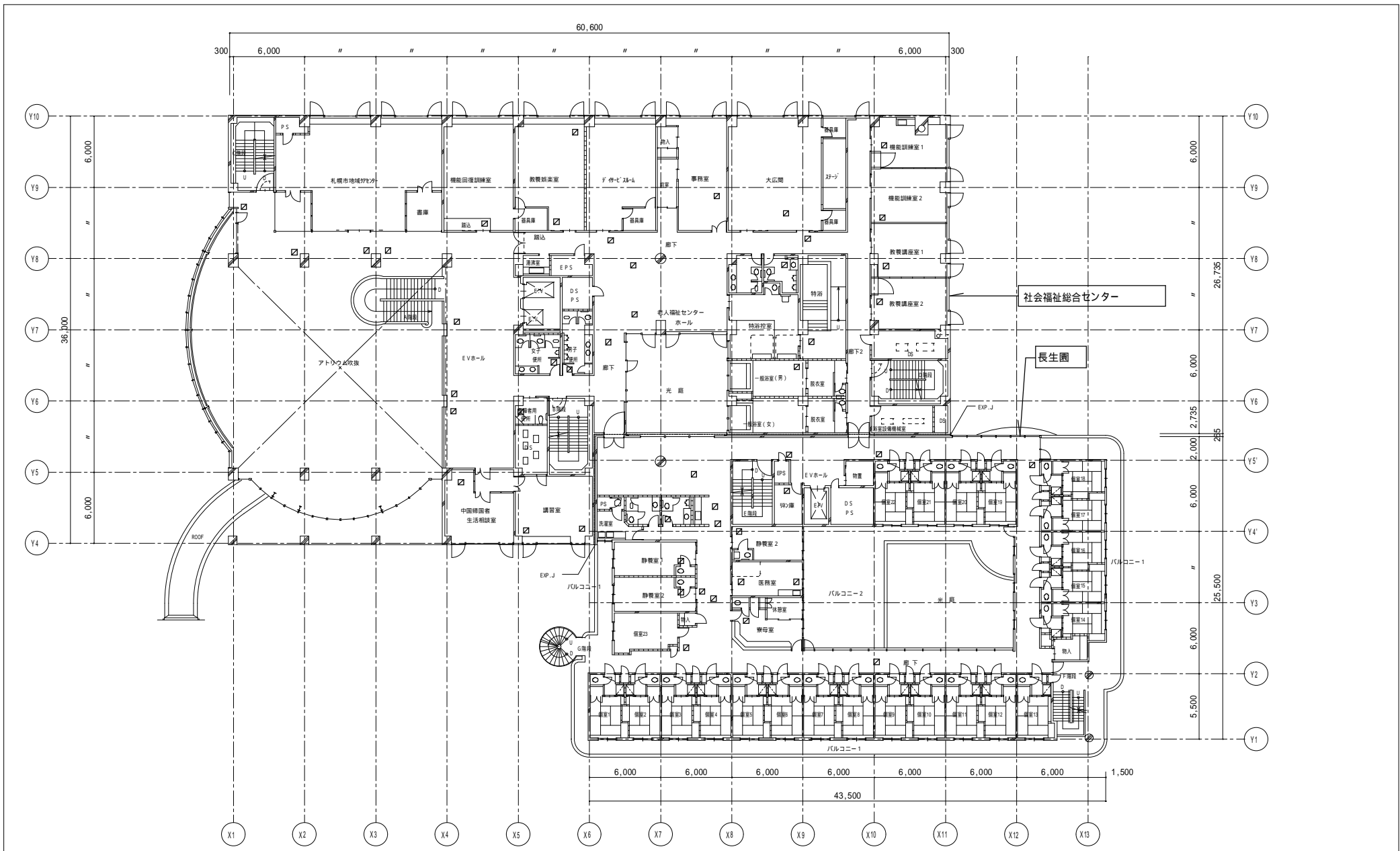
2階平面図 1:300
