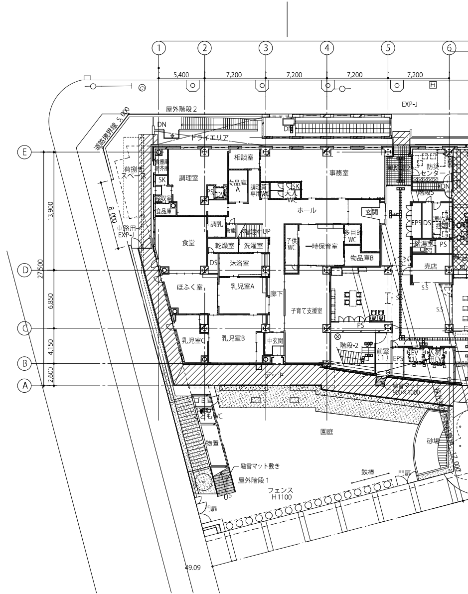
1階平面図 1/300 (A3)
