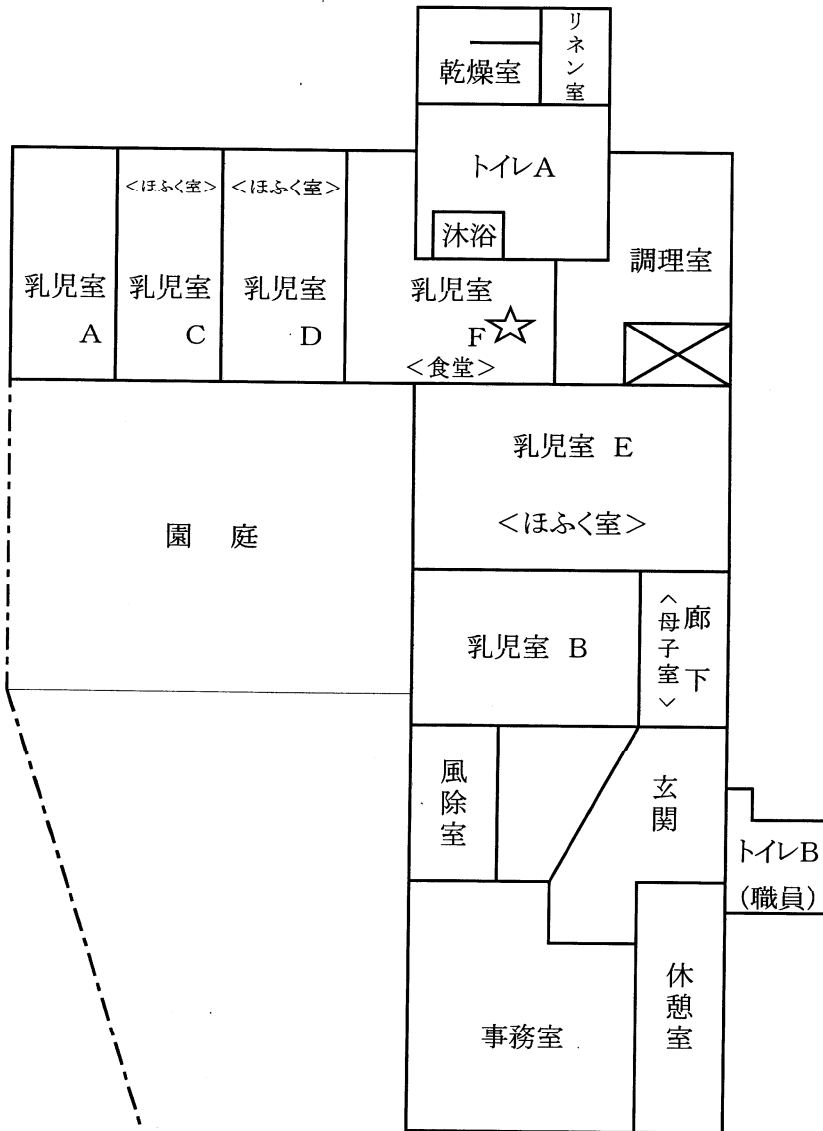
建物の略図
