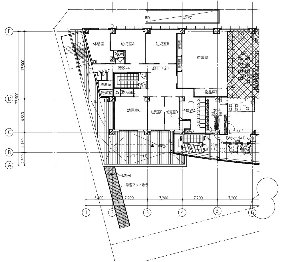
2階平面図 1/300 (A3)
