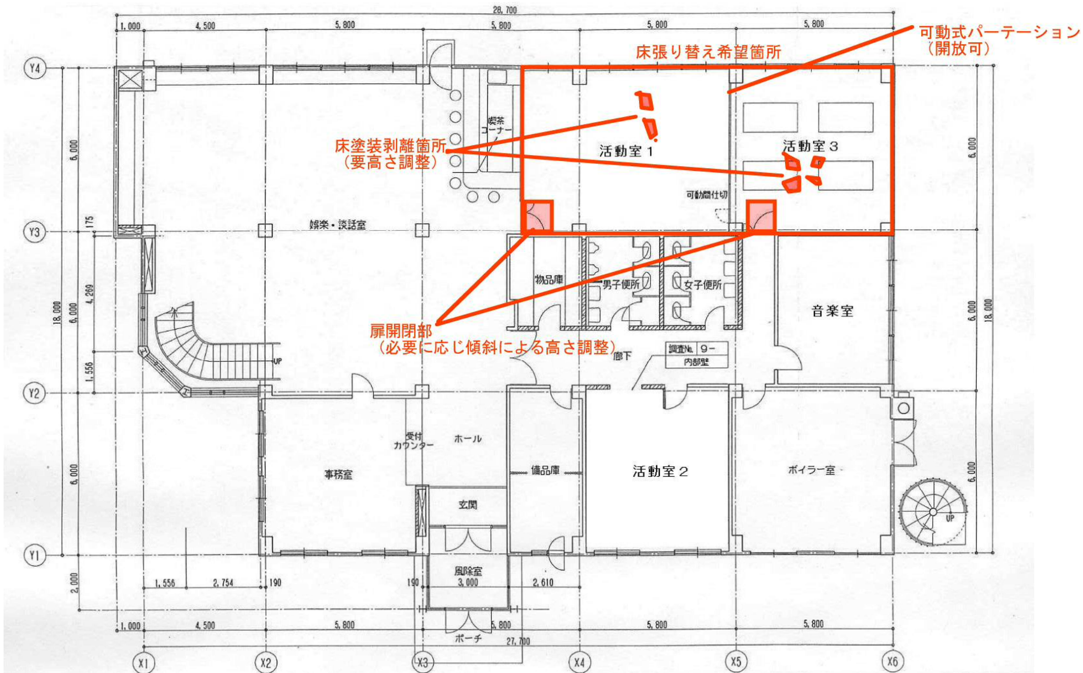
豊平若者活動センター 1階平面図
