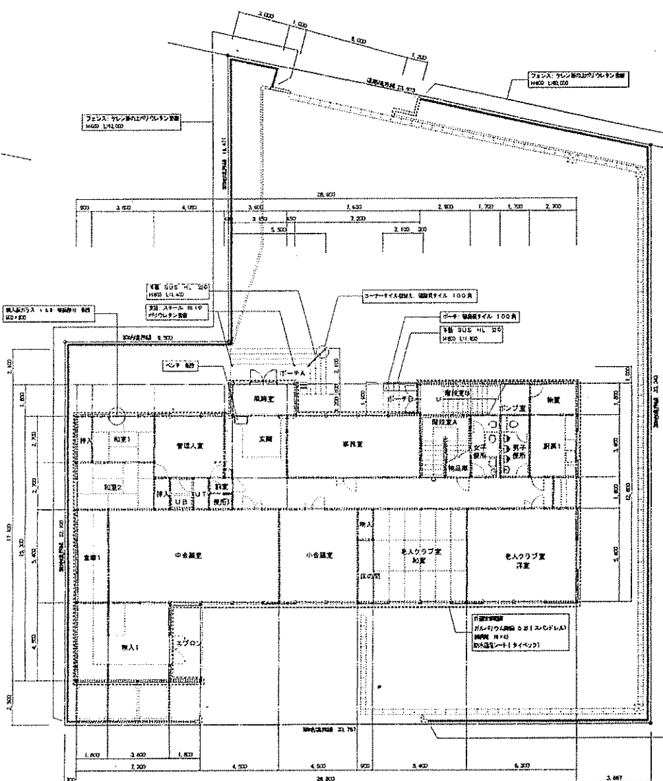
改修 1 階平面図
