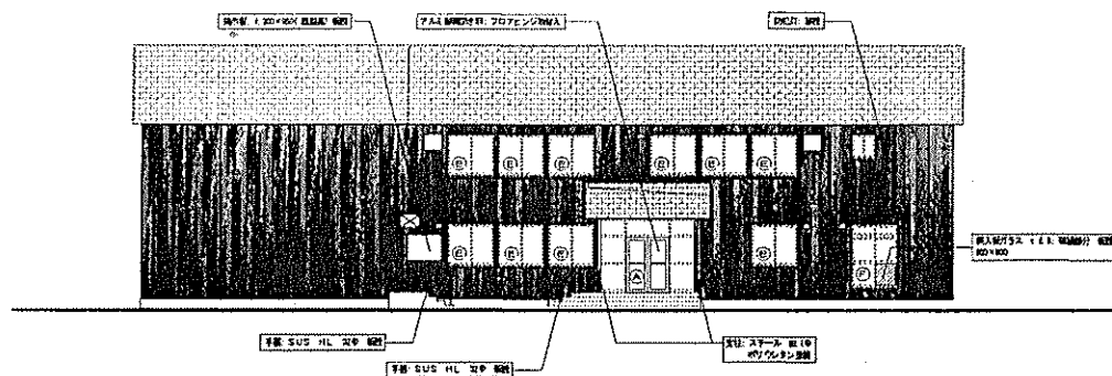
改修 北側立面図
