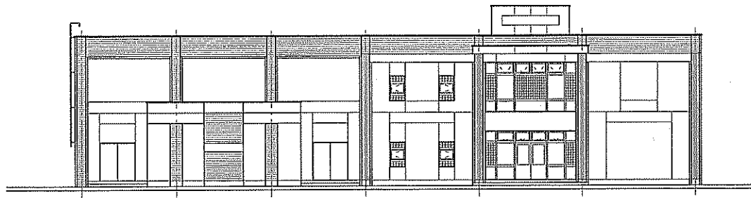
(東 立面图 S=1:100)
