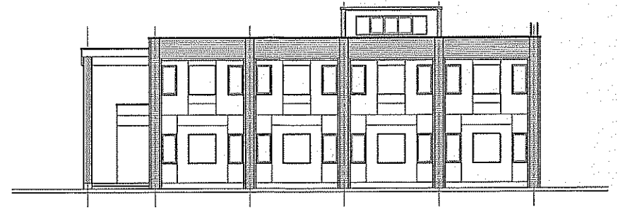
(北 立面图 S=1:100)
