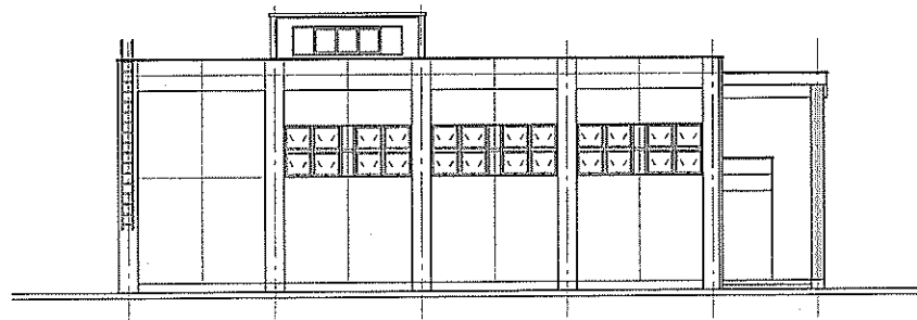
(南 立面图 S=1:100)
