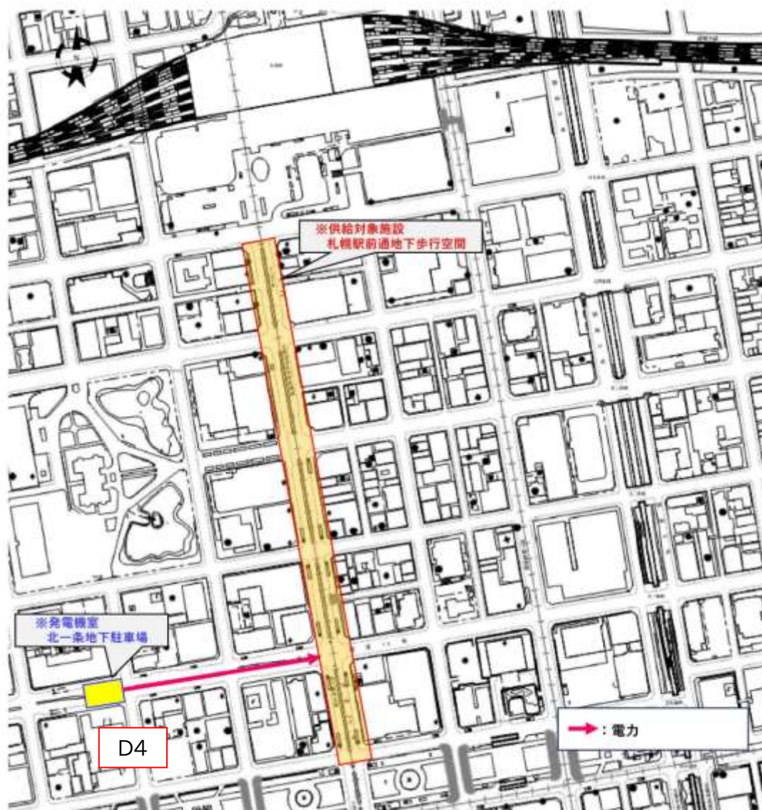
図 18 札幌駅前通地下歩行空間 非常用発電設備 D4 詳細図
