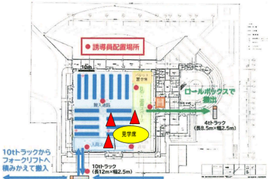
物資集積拠点のレイアウト・車両動線図（屋内）
