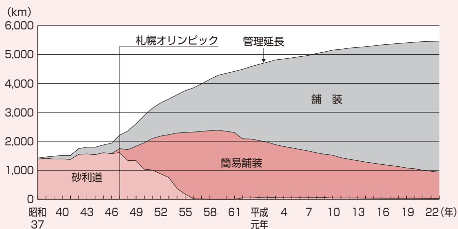
図2-2 道路延長及び舗装状況の推移
