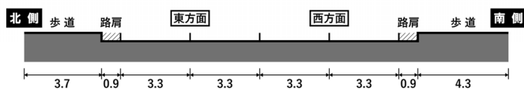
図8.1.1-10(1) 道路断面
