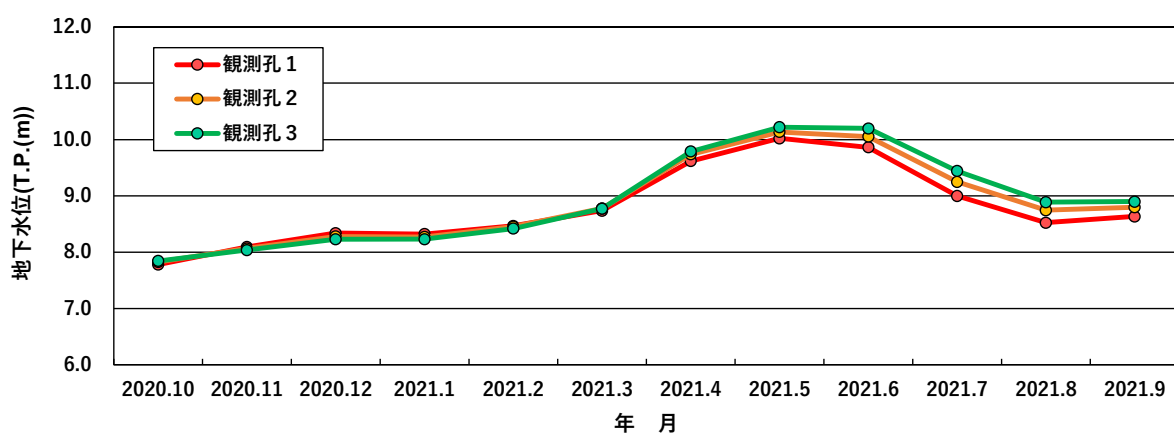
図8.1.6-7(2) 現地調査による地下水の水位の状況(地下水位(月平均値))
