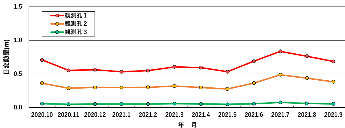
図8.1.6-7(3) 現地調査による地下水の水位の状況(地下水位の日変動量(月平均値))
