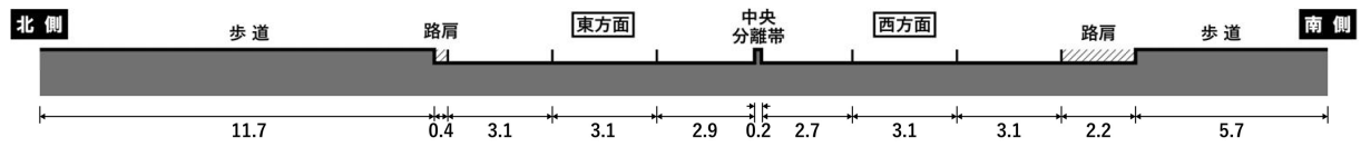
図8.1.1-10(3) 道路断面
