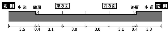
図8.1.1-10(2) 道路断面
