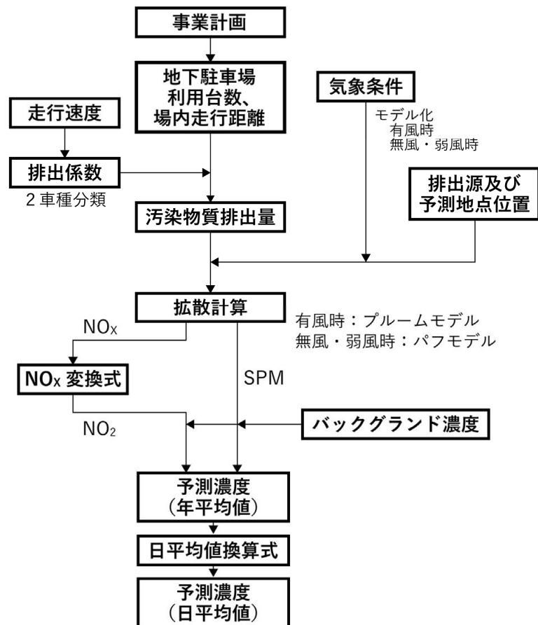
図7.2.1-4 大気汚染物質の濃度の予測手順(地下駐車場の供用)
