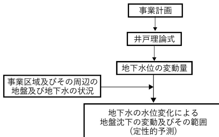
図7.2.6-3 供用後の地盤沈下又は地下水位の変動及びその範囲の予測手順
