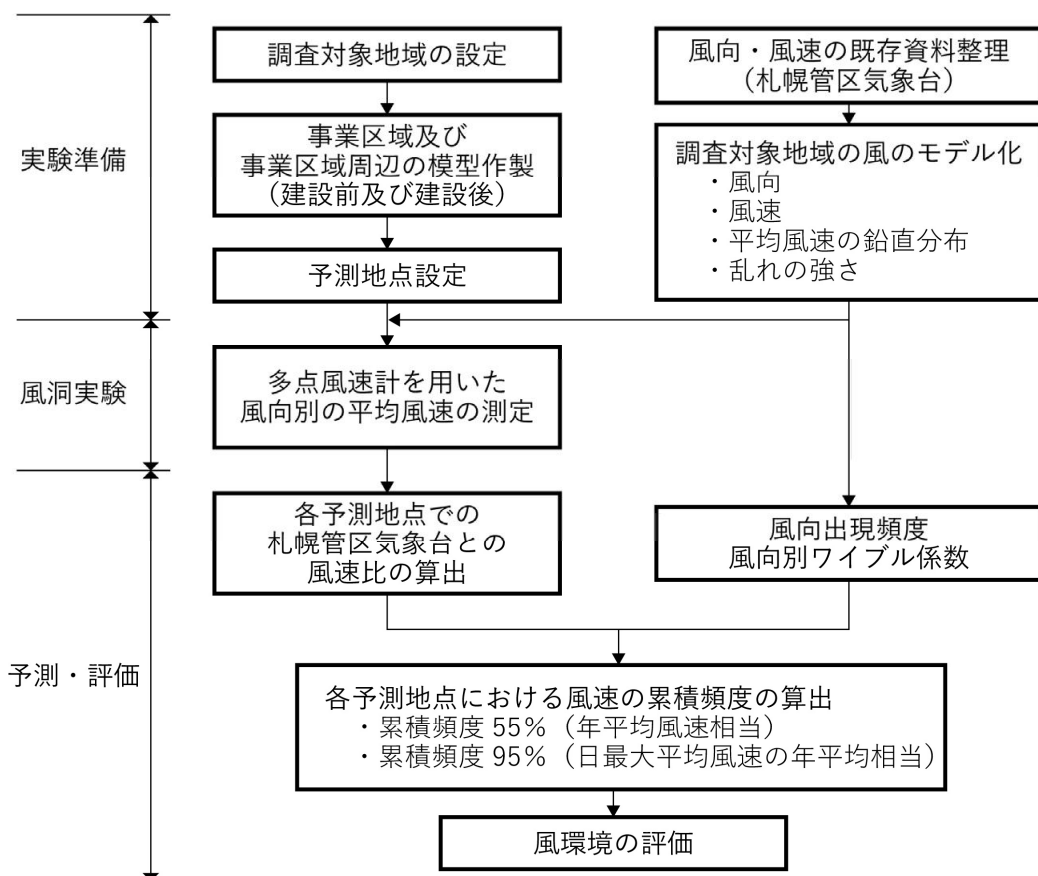
図7.2.4-1 風環境の変化の予測手順
