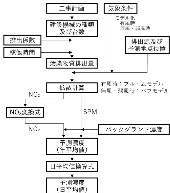
図7.2.1-2 大気汚染物質の濃度の予測手順(建設機械の稼働)
