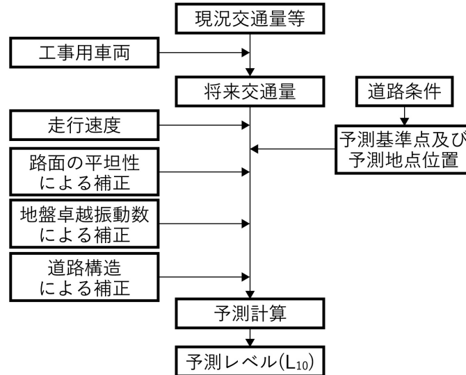
図7.2.3-2 振動レベルの予測手順(工事用車両の運行)
