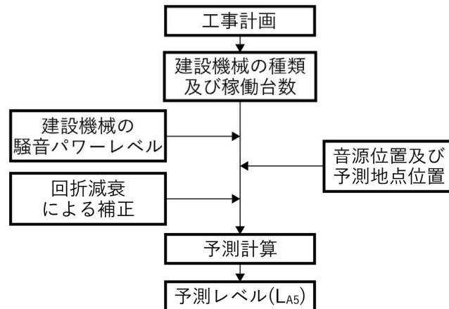
図7.2.2-2 騒音レベルの予測手順(建設機械の稼働)
