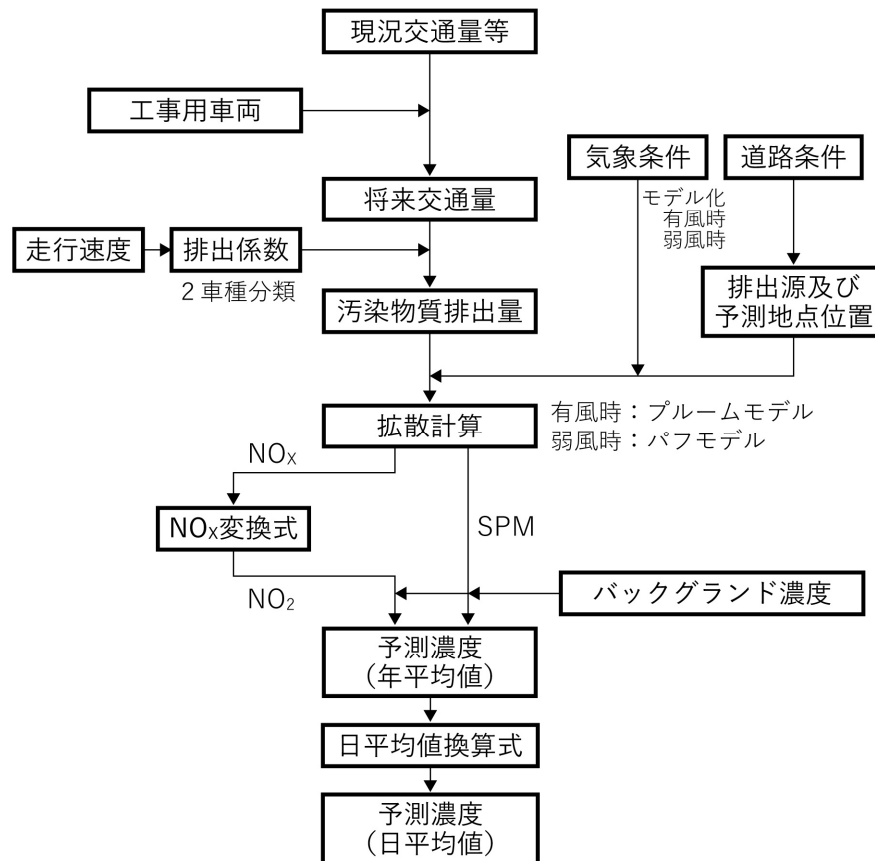
図7.2.1-3 大気汚染物質の濃度の予測手順(工事用車両の運行)
