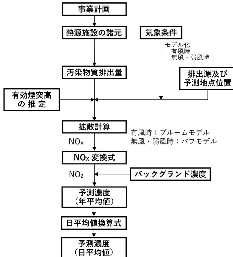
図7.2.1-5 大気汚染物質の濃度の予測手順(地域冷暖房施設の稼働)
