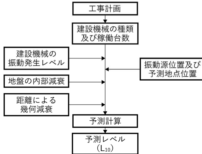
図7.2.3-1 振動レベルの予測手順(建設機械の稼働)
