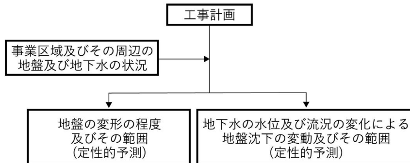
図7.2.6-2 工事中の地盤沈下の変動及びその範囲の予測手順
