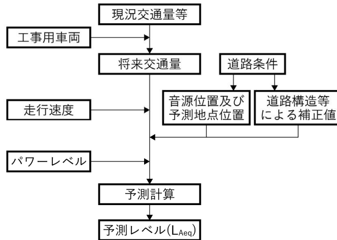
図7.2.2-3 騒音レベルの予測手順(工事用車両の運行)
