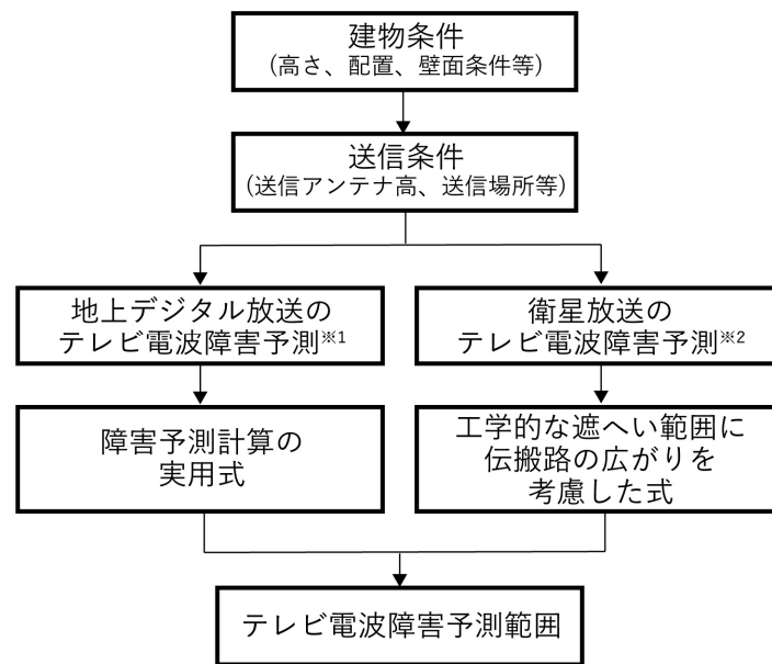
図9.2.8-1 電波障害の予測手順
